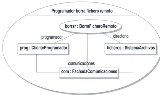
Figura 12.17. Uso de la colaboración para el borrado de un fichero en el servidor
