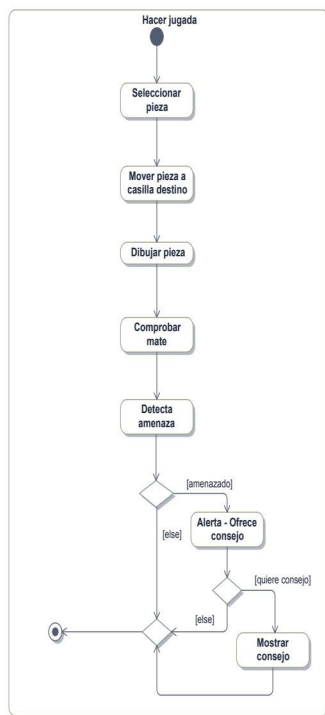
Figura 11.23. Diagrama de actividades para el caso de uso “Hacer jugada”
