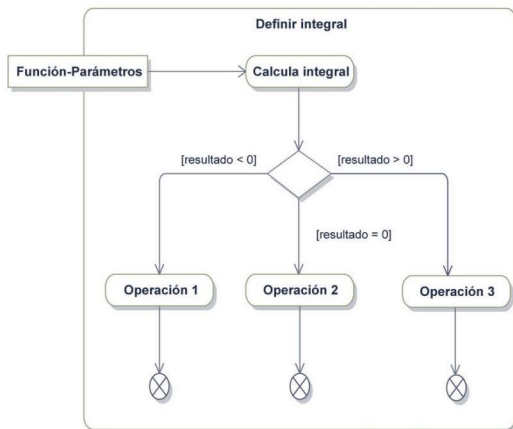
Figura 11.19. Varios flujos a partir de un nodo condicional (al finalizar un flujo los otros no se alteran)
