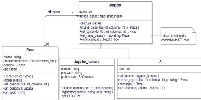
Figura 12.11. Diagrama de clases relacionado con la clase Jugador_humano
