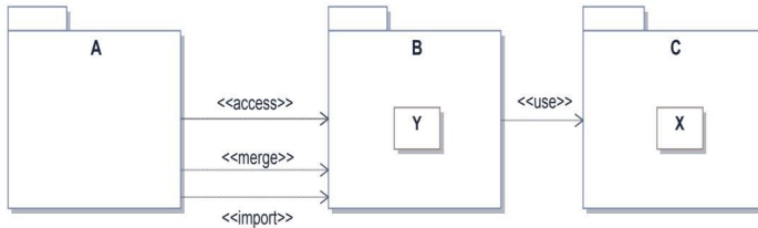
Figura 5.21. Diversos modos de dependencia entre paquetes
