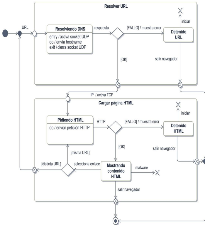
Figura 10.11. Ejemplo de estado compuesto simple
