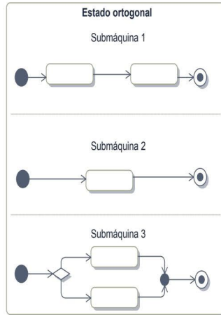
Figura 10.12. Estado compuesto ortogonal (3 submáquinas)
