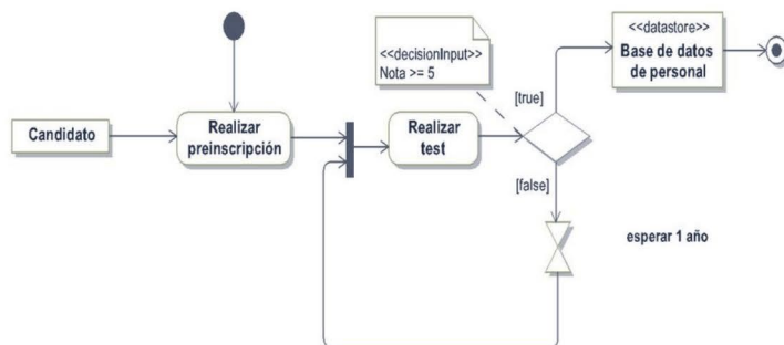
Figura 11.7. Ejemplo de uso de un nodo de datos
