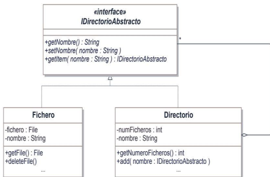
Figura 9.31. Aplicación del patrón Composite
