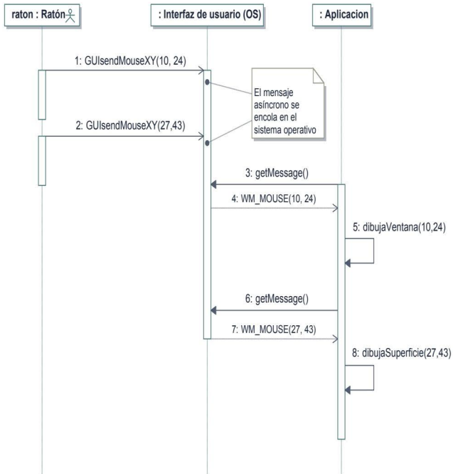
Figura 7.5. Ejemplo de mensajes asíncronos
