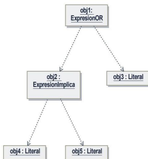
Figura 9.26. Distribución de los objetos en memoria
