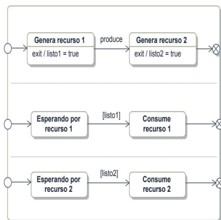
Figura 10.14. Tres submáquinas concurrentes con sincronización
