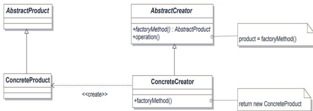
Figura 9.9. Estructura del patrón Factory Method
