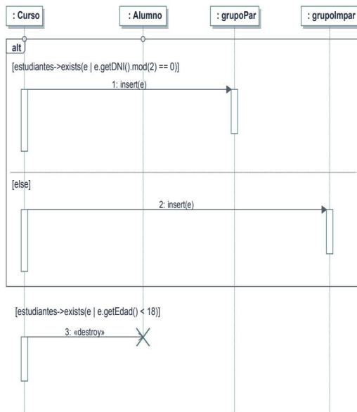
Figura 13.6. Diagrama de secuencias para inclusión de alumno en grupo
