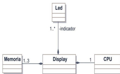
Figura 6.12. Ejemplo de composición
