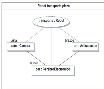
Figura 12.10. Diagrama de uso de colaboración de la figura 12.9
