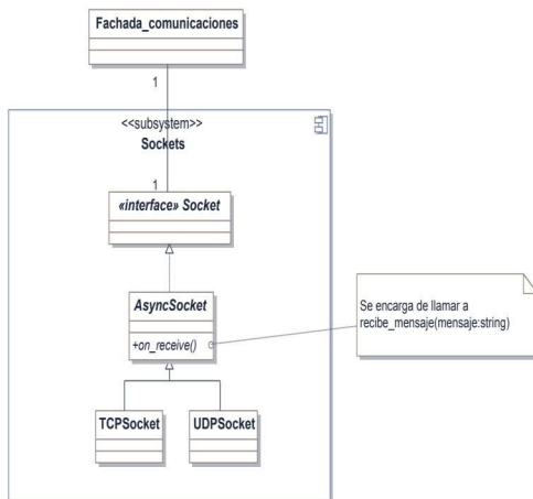
Figura 9.27. Aplicación del patrón Facade
