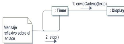
Figura 8.3. Ejemplo de mensaje reflexivo
