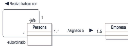
Figura 6.9. Relación reflexiva de la clase Persona
