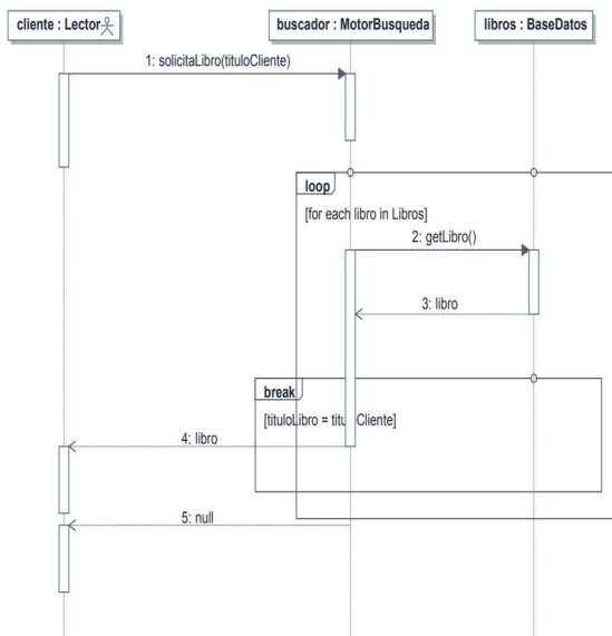
Figura 14.17. Diagrama de secuencias con fragmento iterativo
