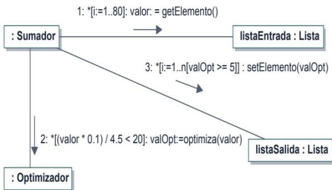
Figura 8.6. Ejemplo de iteraciones y condicionales
