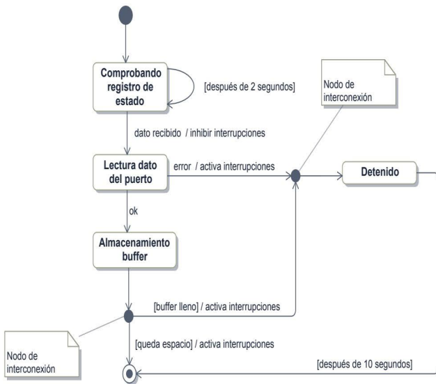
Figura 10.6. Ejemplo de diagrama con nodos de interconexión
