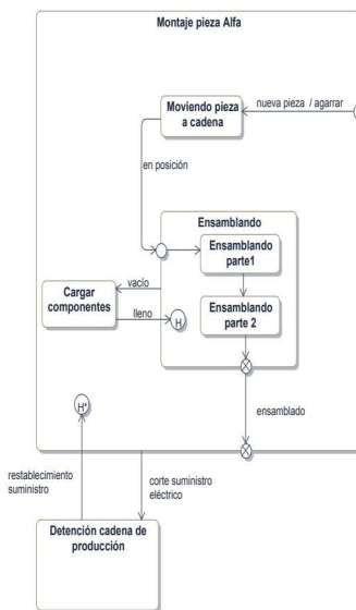
Figura 10.18. Ejemplo de uso de los dos tipos de nodos de historial (H y H*)
