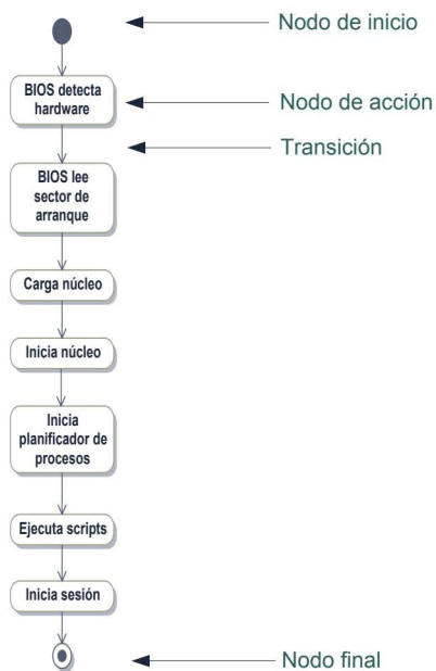
Figura 11.1. Ejemplo básico de un diagrama de actividad
