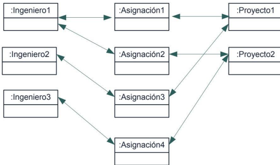
Figura 6.8. Asignación entre pares de objetos (diagrama de objetos)
