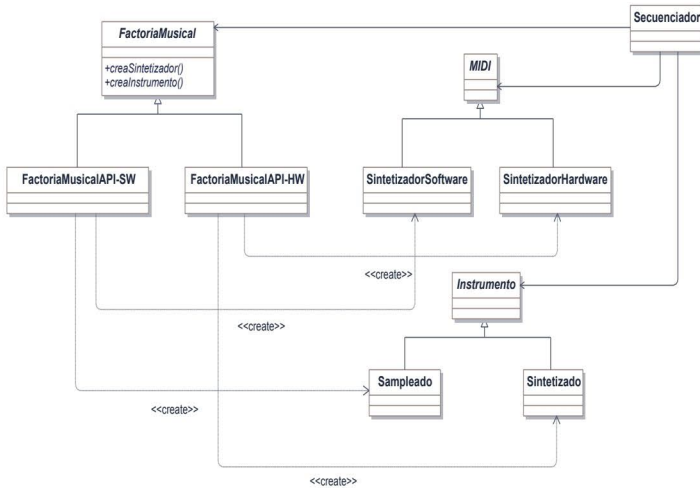
Figura 9.5. Ejemplo del patrón Abstract Factory
