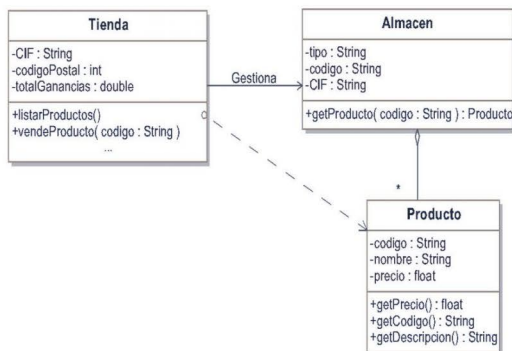
Figura 6.16. Ejemplo de dependencia entre la clase Tienda y la clase Producto
