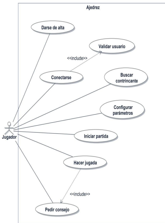
Figura 2.4. Diagrama ampliado para el juego del ajedrez
