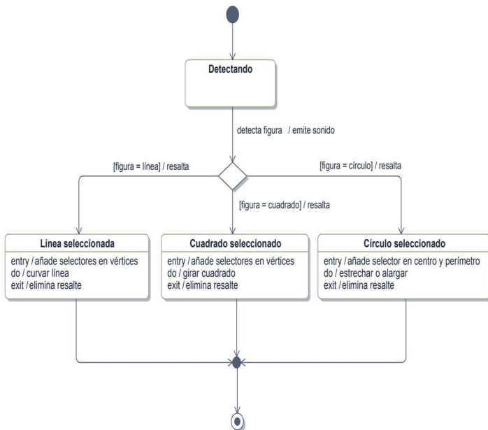
Figura 10.7. Utilización del nodo condicional
