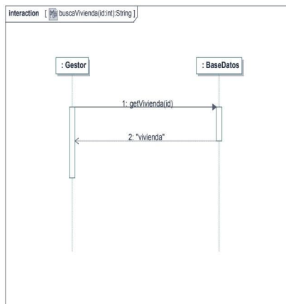
Figura 7.15. Diagrama de secuencias invocado
