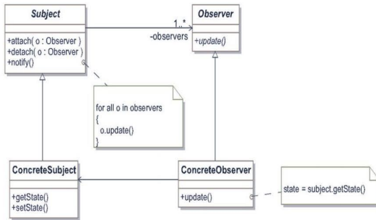
Figura 9.17. Estructura del patrón Observer
