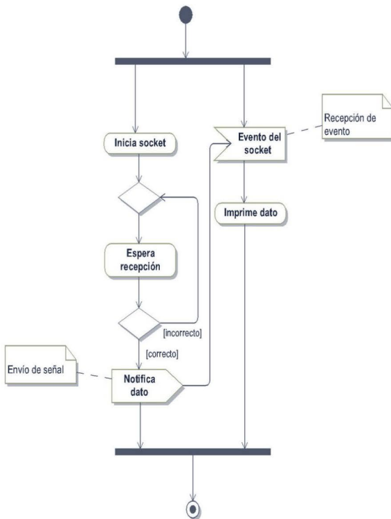
Figura 11.18. Ejemplo de señal y evento
