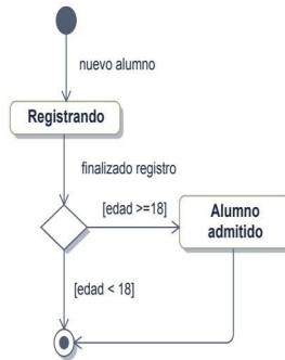
Figura 13.7. Diagrama de estados del proceso de matriculación
