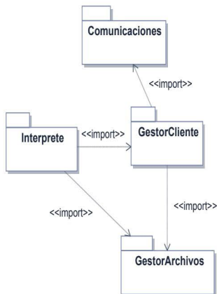
Figura 5.23. Diagrama de paquetes para la aplicación Mercurial en versión Java
