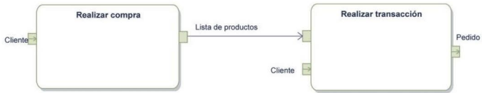
Figura 11.10. Ejemplo de dos actividades interconectadas por pines
