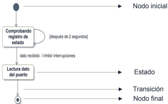
Figura 10.5. Diagrama de estados elemental
