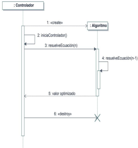
Figura 7.6. Creación de objeto, invocación recursiva y destrucción de objeto
