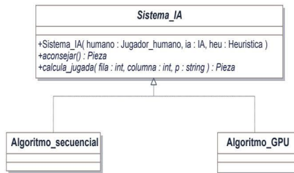
Figura 9.29. Aplicación del patrón Strategy
