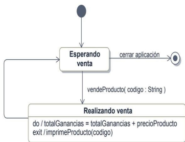
Figura 10.9. Diagrama de estados con eventos de llamada
