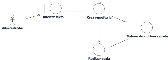
Figura 3.9. Diseño de robustez del caso de uso “Clonar repositorio” de Mercurial
