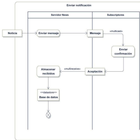
Figura 11.22. Ejemplo de <<multicast>> y <<multireceive>>
