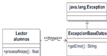
Figura 6.17. Ejemplo de uso de excepciones
