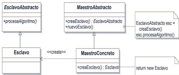
Figura 9.10. Ejemplo del patrón Factory Method
