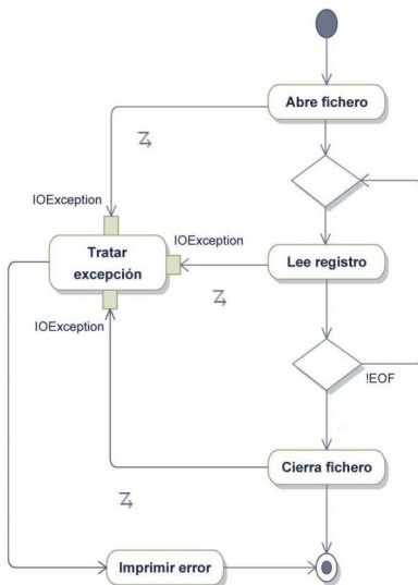
Figura 11.16. Lectura de fichero y contexto de manejo de excepciones
