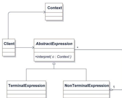
Figura 9.24. Estructura del patrón Interpreter
