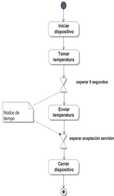
Figura 11.5. Diagrama con dos eventos de tiempo
