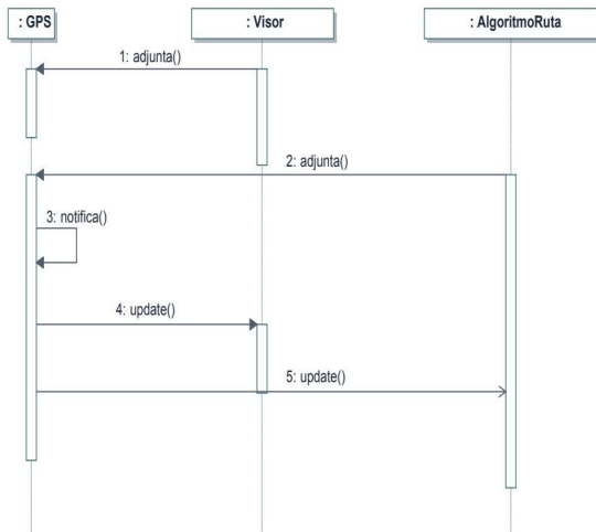
Figura 9.19. Diagrama de secuencias del ejemplo anterior
