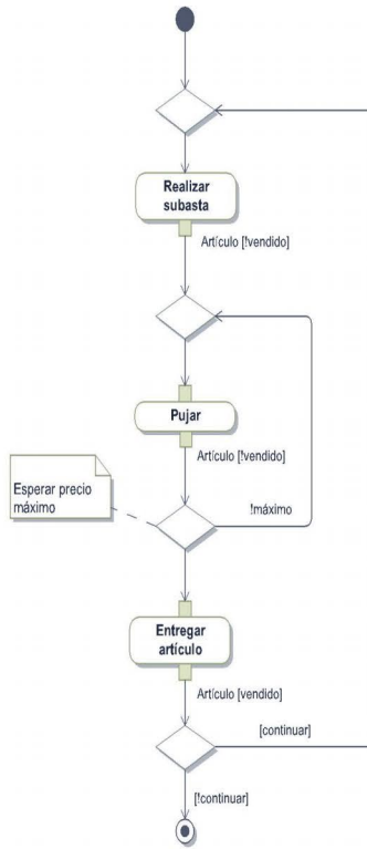
Figura 11.11. Ejemplo de pines con estado
