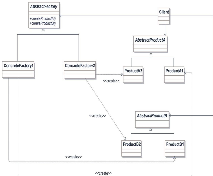
Figura 9.4. Estructura del patrón Abstract Factory
