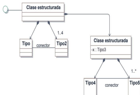
Figura 12.1. Diagrama de clases de ejemplo
