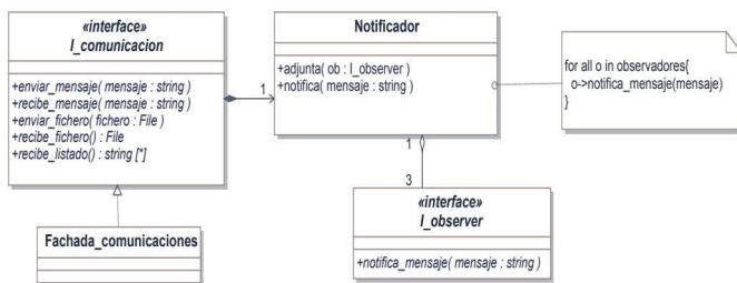
Figura 9.28. Aplicación del patrón Observer
