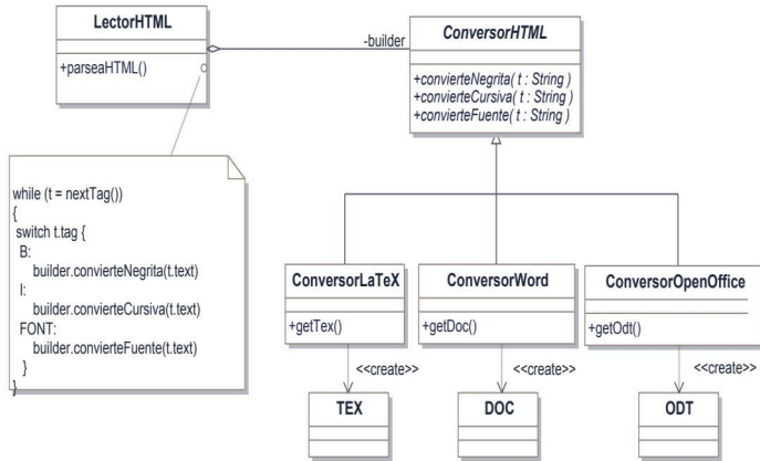
Figura 9.7. Ejemplo del patrón Builder
