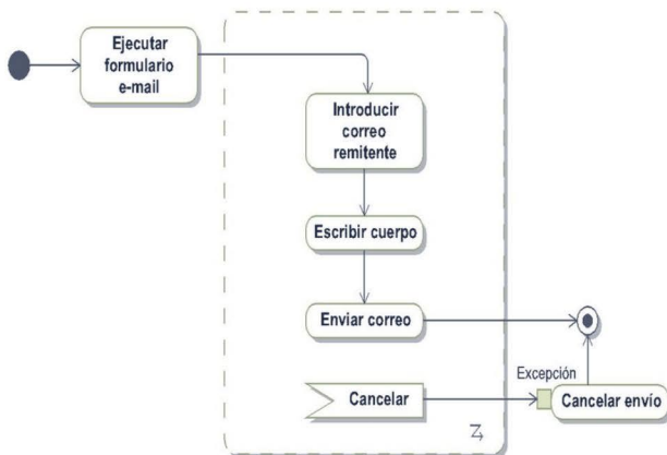
Figura 11.13. Ejemplo de región interrumpible en un formulario Web
