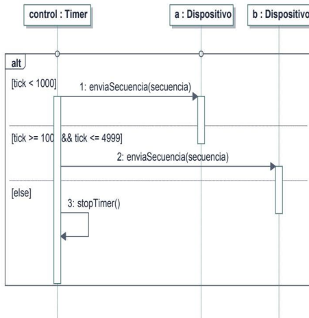
Figura 14.16. Diagrama de secuencias con fragmento condicional
