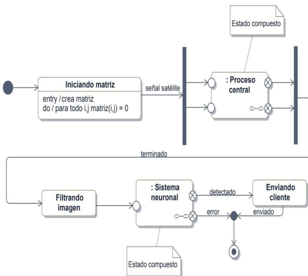
Figura 10.15. Simplificación de la figura 10.13 utilizando iconos de estado compuesto
