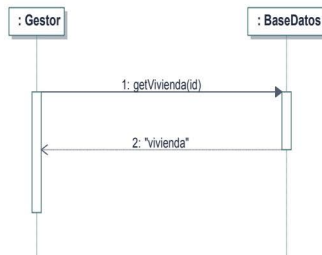
Figura 15.13. Diagrama de secuencias
