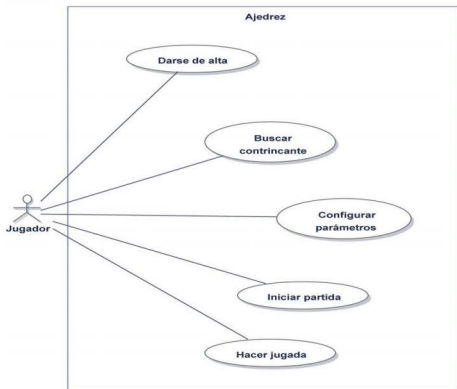
Figura 2.3. Ejemplo de diagrama de casos de uso para el juego de ajedrez
