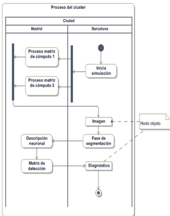
Figura 11.8. Ejemplo de actividad partida
