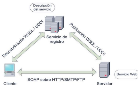
Figura 9.2. Arquitectura de un Servicio Web
