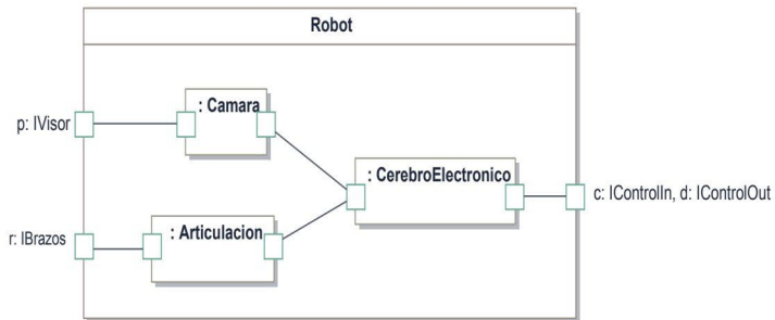
Figura 12.7. Diagrama de estructura compuesta con varios puertos
