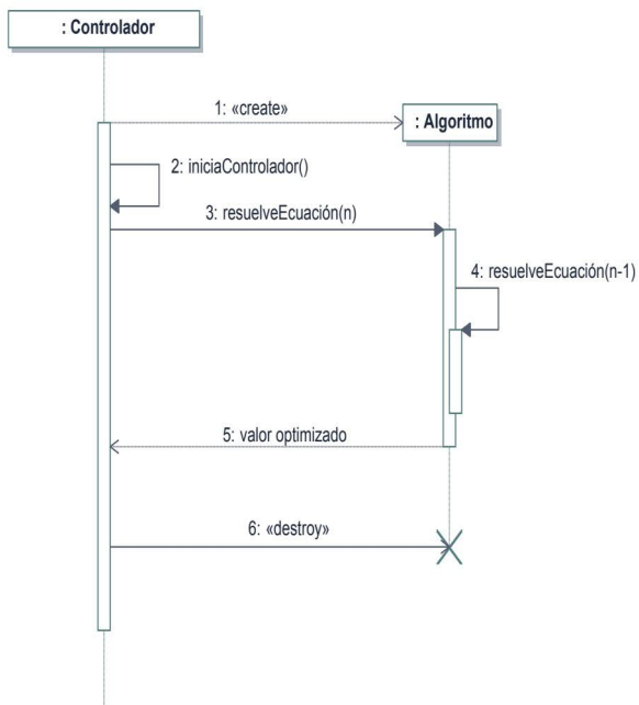
Figura 14.15. Diagrama de secuencias de un controlador que solicita una optimización
