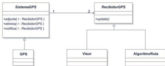
Figura 9.18. Ejemplo de patrón Observer
