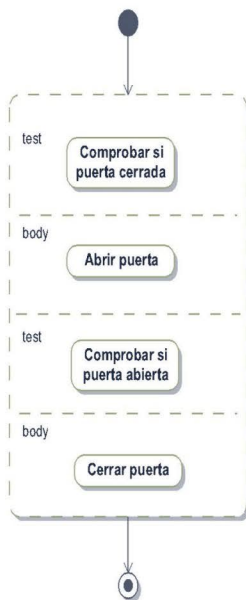
Figura 11.14. Ejemplo de región if
