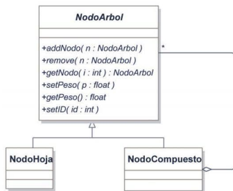
Figura 9.12. Ejemplo de patrón Composite
