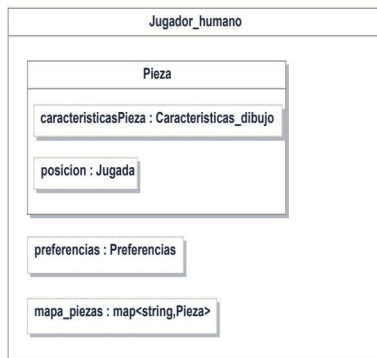
Figura 12.12. Diagrama de estructura compuesta para la clase Jugador_humano
