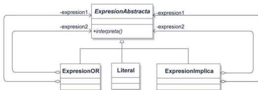
Figura 9.25. Ejemplo del patrón Interpretador
