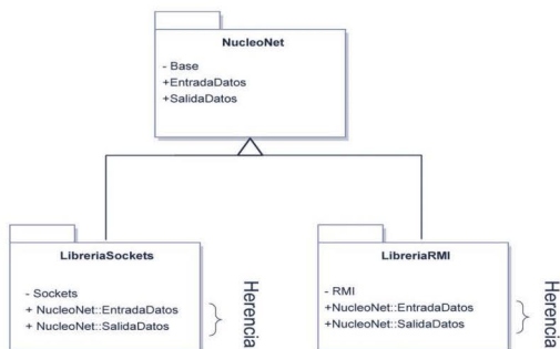
Figura 5.20. Ejemplo de generalización
