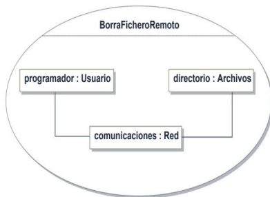
Figura 12.16. Diagrama de colaboración para la clase Usuario
