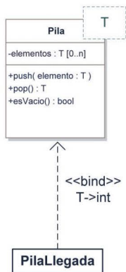
Figura 6.18. Clase Plantilla y enlace al tipo concreto mediante <<bind>>
