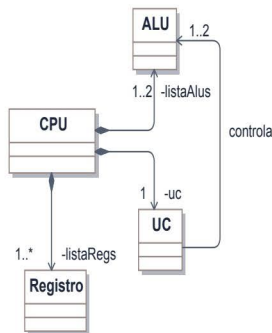
Figura 14.9. Ejemplo de composición
