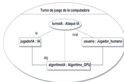
Figura 12.14. Uso de colaboración para el ataque de la computadora
