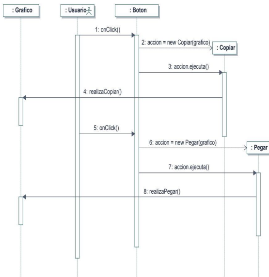
Figura 9.16. Diagrama de secuencias del ejemplo anterior
