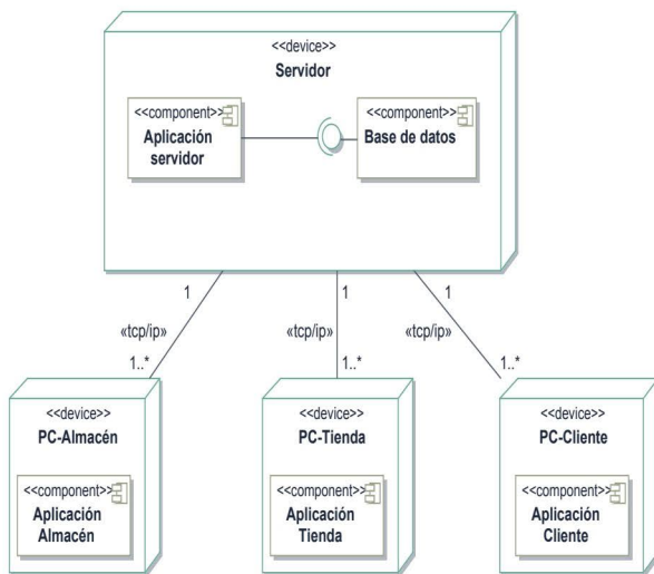
Figura 5.14. Ejemplo de diagrama de despliegue con varios nodos y componentes
