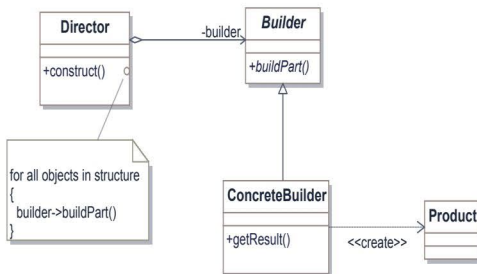
Figura 9.6. Estructura del patrón Builder
