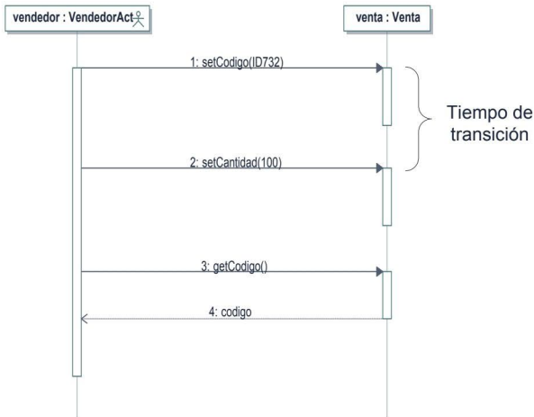
Figura 7.3. Diagrama de secuencias de una venta
