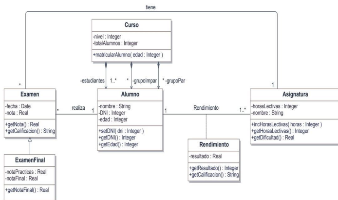
Figura 13.1. Diagrama de clases para una academia
