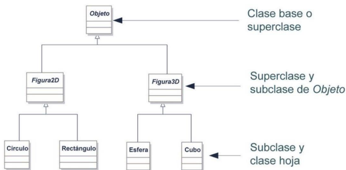
Figura 6.13. Herencia (los nombres de las clases abstractas se escriben en cursiva)
