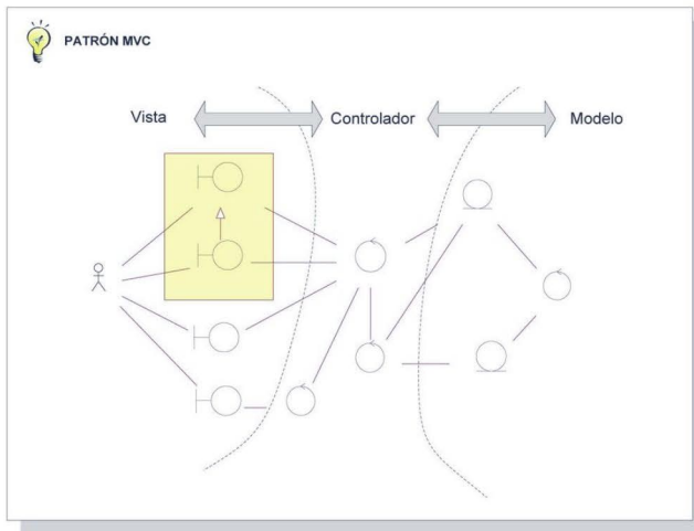
Figura 3.4. Los casos de uso de la aplicación ajedrez se adecuan al patrón MVC
