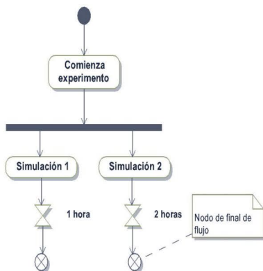
Figura 11.20. Dos flujos concurrentes finalizados independientemente
