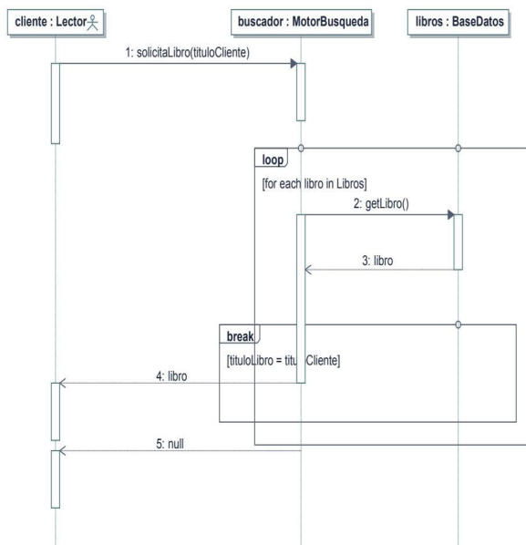
Figura 7.12. Terminación de bucle con break
