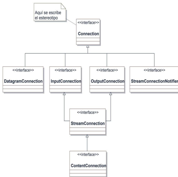
Figura 6.15. Jerarquía de interfaces en una de las librerías de Java
