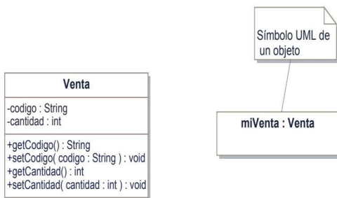
Figura 7.1. Ejemplo de clase (izquierda) e instancia de la misma (derecha)
