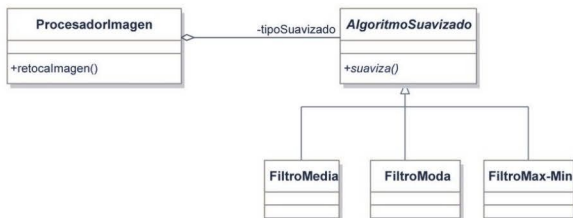
Figura 9.21. Ejemplo del patrón Strategy
