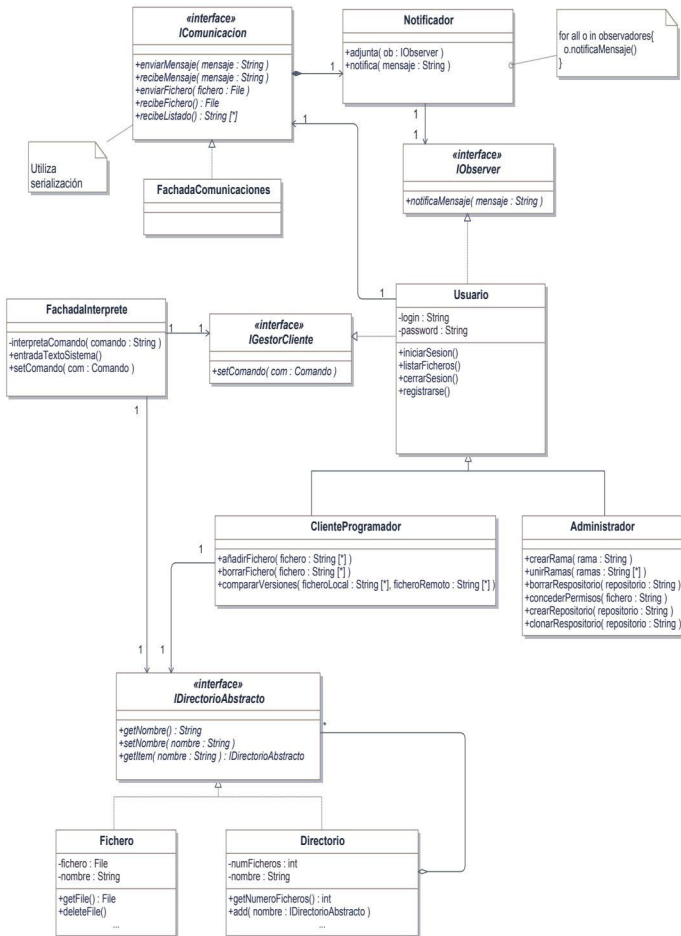
Figura 6.22. Diagrama de clases de Mercurial
