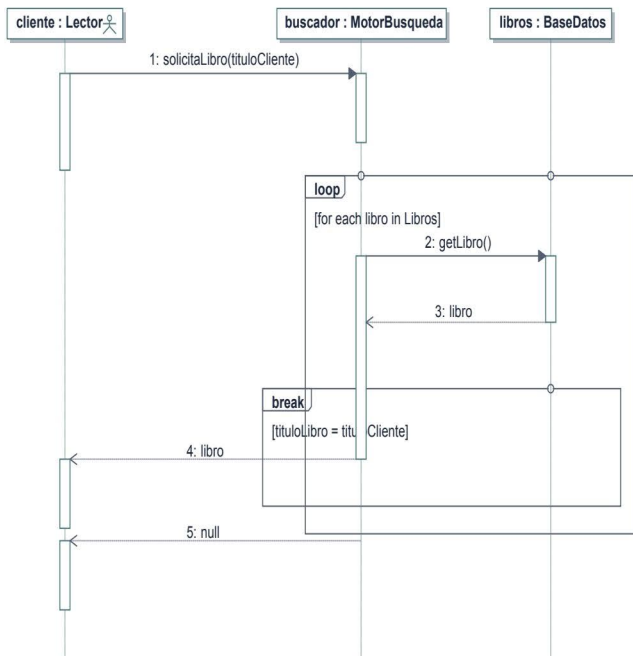
Figura 15.16. Diagrama de secuencias con fragmento iterativo
