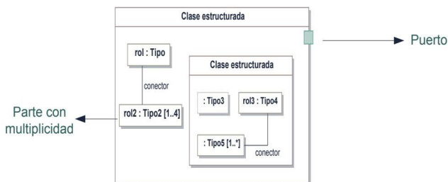
Figura 12.2. Diagrama de estructura compuesta correspondiente a la figura 12.1
