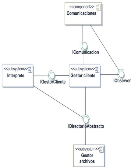
Figura 5.12. Diagrama de componentes para la aplicación Mercurial
