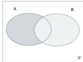
Figura 13.4. Diferencia (A - B)
