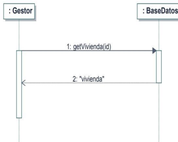
Figura 7.4. Mensajes síncronos
