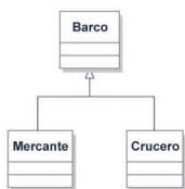
Figura 15.5. Simple
