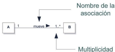
Figura 4.2. Asociación
