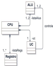
Figura 15.9. Composición
