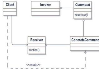
Figura 9.14. Estructura del patrón Command
