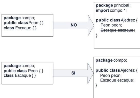
Figura A.1. Ejemplo de importación con paquetes
