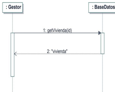
Figura 14.14. Diagrama de secuencias
