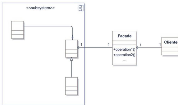
Figura 9.13. Estructura del patrón Facade
