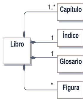
Figura 4.6. Ejemplo de composición
