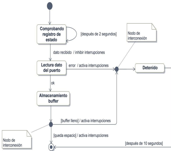
Figura 15.17. Diagrama de estado del procesamiento de un dato por un manejador de dispositivo
