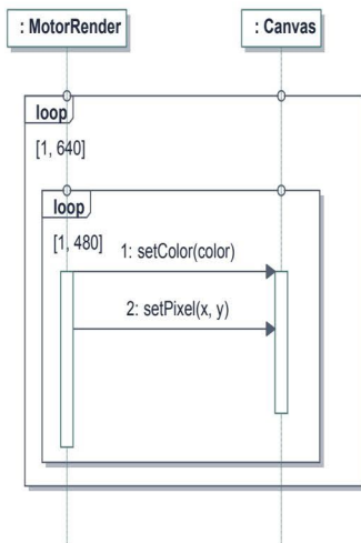
Figura 7.11. Ejemplo de bucle anidado
