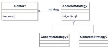
Figura 9.20. Estructura del patrón Strategy
