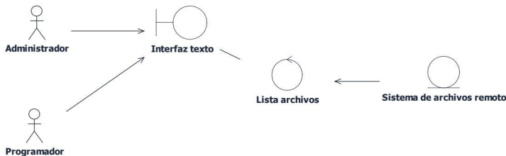
Figura 3.8. Diagrama de robustez para el caso de uso “Listar ficheros” de Mercurial
