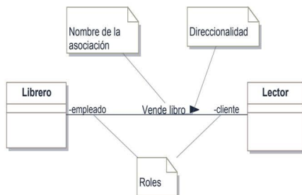
Figura 6.4. Ejemplo de una asociación con navegabilidad simétrica
