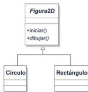
Figura 15.10. Ejemplo de clase abstracta con herencia
