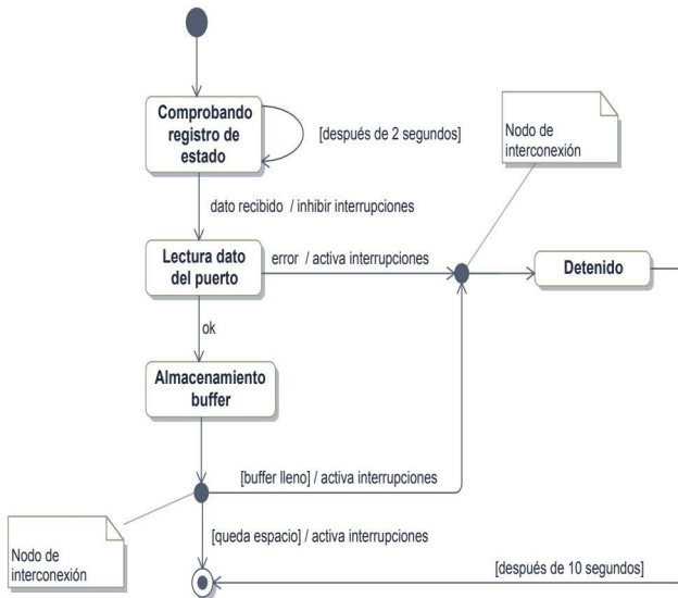
Figura 14.18. Diagrama de estado del procesamiento de un dato por un manejador de dispositivo
