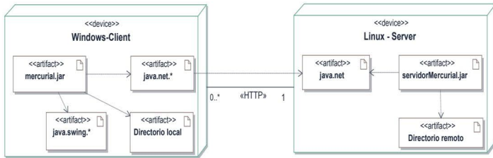
Figura 5.16. Diagrama de despliegue para Mercurial en versión Java
