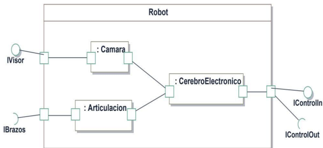
Figura 12.8. Clase estructurada con puerto explícito
