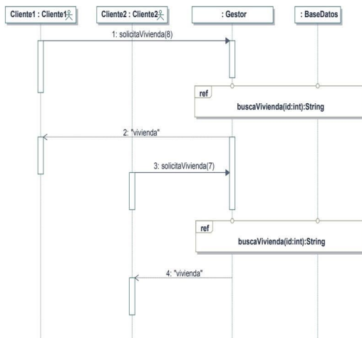
Figura 7.14. Llamada a otro diagrama de secuencias
