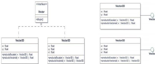
Figura 6.14. Dos representaciones de la interfaz Vector
