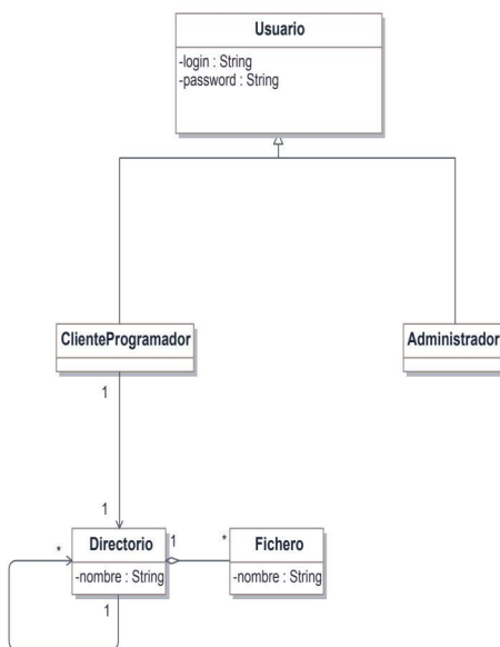
Figura 4.12. Modelo del dominio para Mercurial
