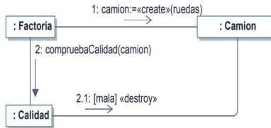
Figura 8.4. Ejemplo de mensajes de "creación" y "destrucción"
