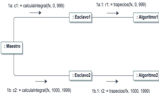
Figura 8.2. Diagrama con situación de concurrencia
