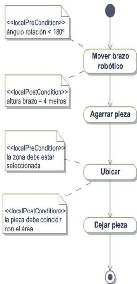
Figura 11.2. Ejemplo de uso de restricciones
