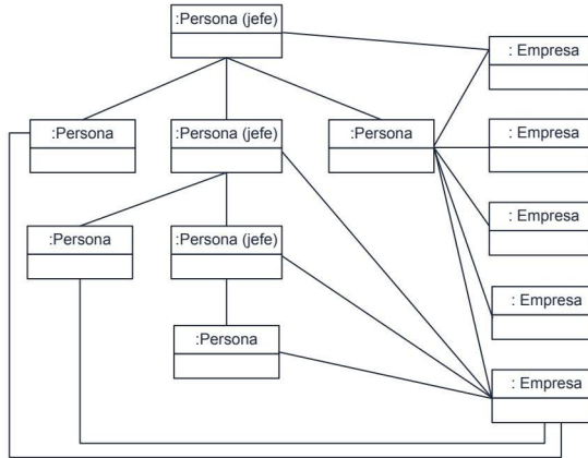
Figura 6.10. Diagrama de objetos de la figura 6.9
