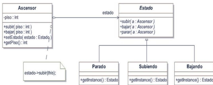
Figura 9.23. Ejemplo del patrón State
