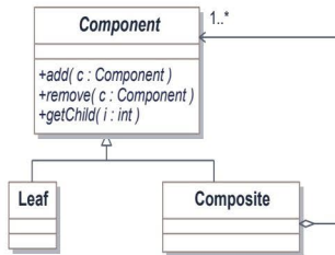
Figura 9.11. Estructura del patrón Composite
