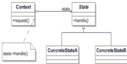
Figura 9.22. Estructura del patrón State
