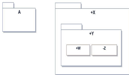
Figura 5.17. Ejemplos de diferentes tipos de paquetes
