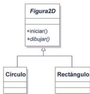
Figura 14.10. Ejemplo de clase abstracta con herencia
