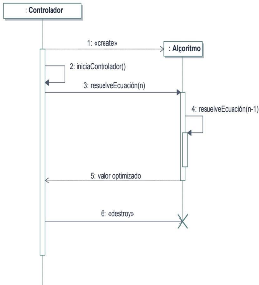
Figura 15.14. Diagrama de secuencias de un controlador que solicita una optimización
