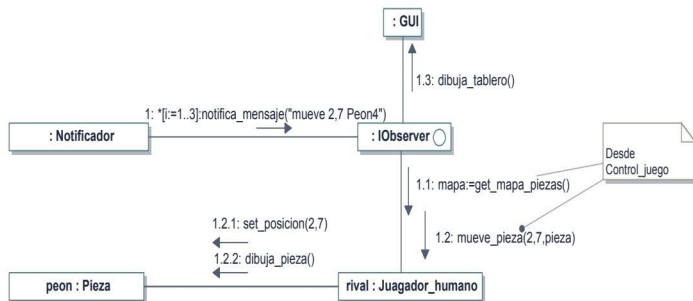
Figura 8.7. Diagrama de comunicación para un movimiento de pieza del rival
