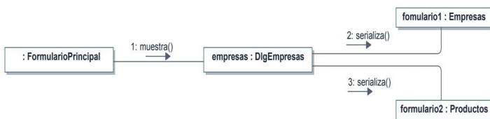
Figura 8.1. Ejemplo de diagrama de comunicación
