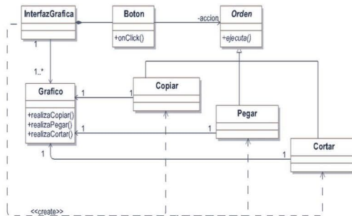
Figura 9.15. Ejemplo del patrón Command
