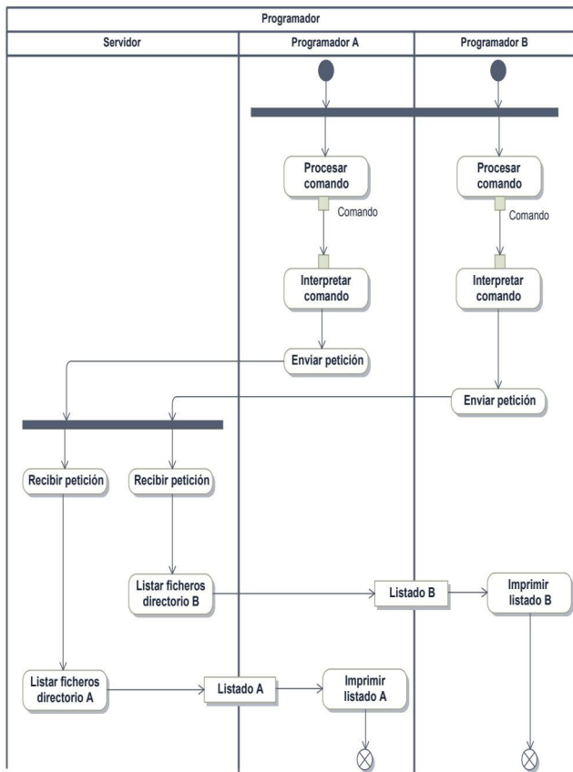
Figura 11.24. Diagrama de actividades para el caso de uso "Listar ficheros"
