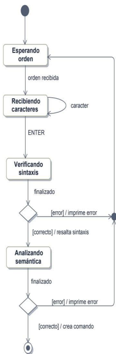
Figura 10.20. Diagrama de estados para procesar un comando en Mercurial
