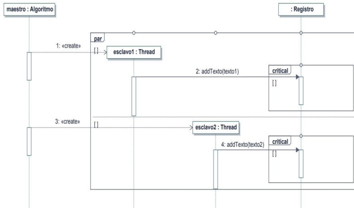
Figura 7.13. Ejemplo de paralelismo con sección crítica
