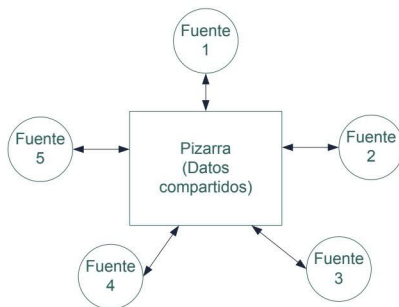
Figura 5.3. Arquitectura de repositorio
