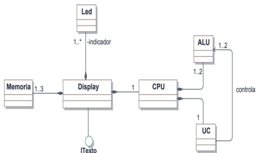
Figura 12.3. Diagrama de clases ampliado de Display
