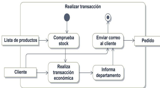
Figura 11.9. Actividad con dos entradas y una salida
