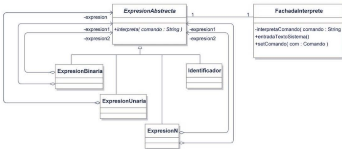
Figura 9.30. Aplicación conjunta de los patrones Facade e Interpreter
