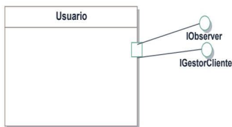
Figura 12.15. Diagrama de estructura compuesta para la clase Usuario
