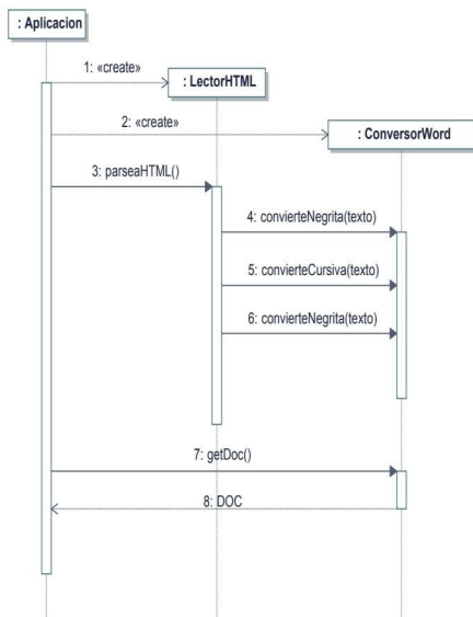
Figura 9.8. Diagrama de secuencias del ejemplo anterior
