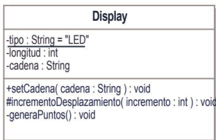
Figura 15.1. Ejemplo de clase en UML
