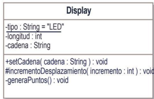
Figura 14.1. Ejemplo de clase en UML
