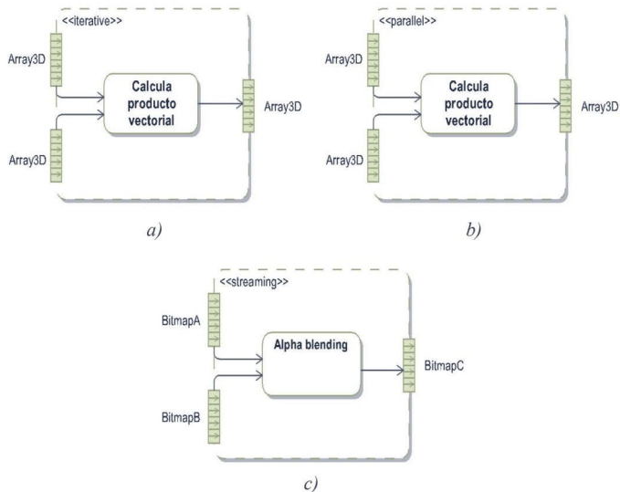
Figura 11.12. Ejemplos de modos de las regiones de expansión
