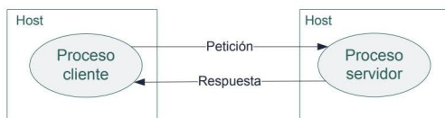
Figura 5.4. Arquitectura cliente-servidor
