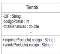
Figura 10.8. Clase Tienda
