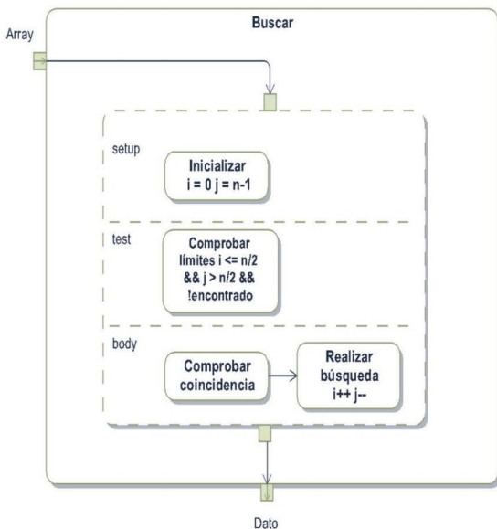
Figura 11.15. Región loop
