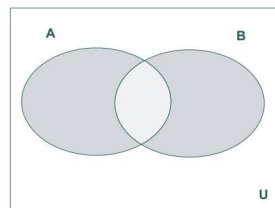
Figura 13.5. Intersección (A \cup B) - (A \cap B)
