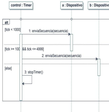
Figura 7.10. Operador alt
