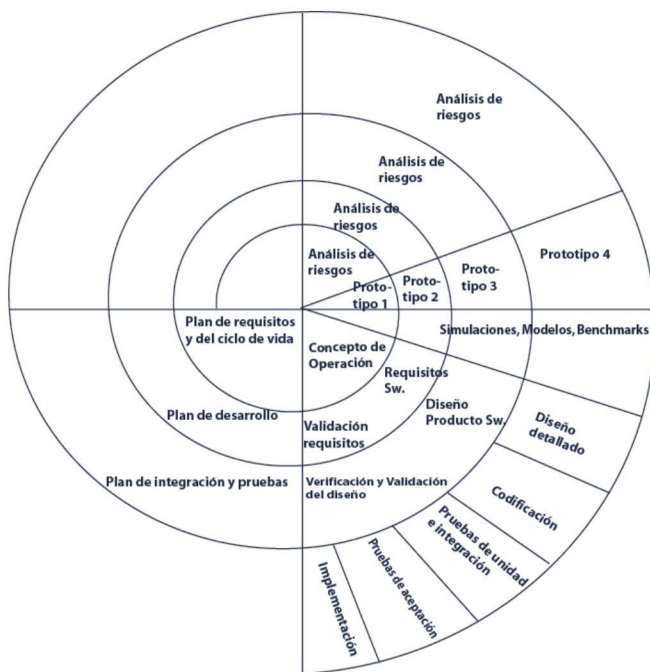
Figura 1.2. Ciclo de vida en espiral
