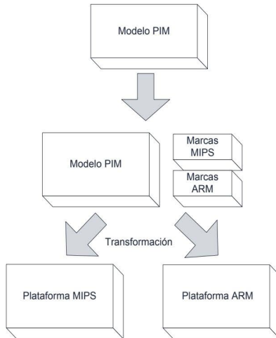
Figura 1.4. Transformación del PIM al PSM
