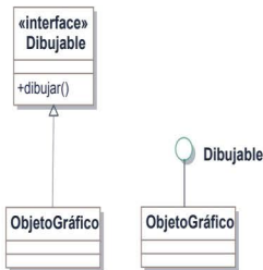
Figura 14.6. Herencia de interface (dos versiones de representación)
