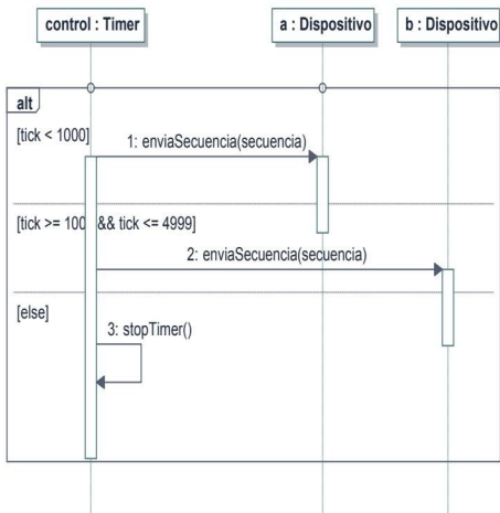
Figura 15.15. Diagrama de secuencias con fragmento condicional
