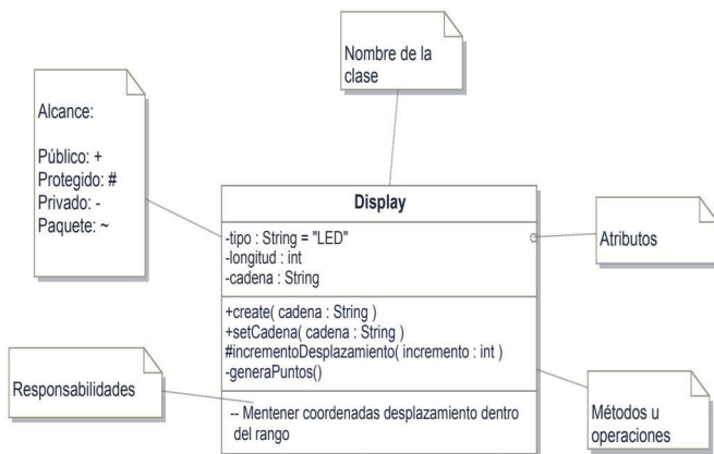
Figura 6.1. Plantilla para una clase en UML
