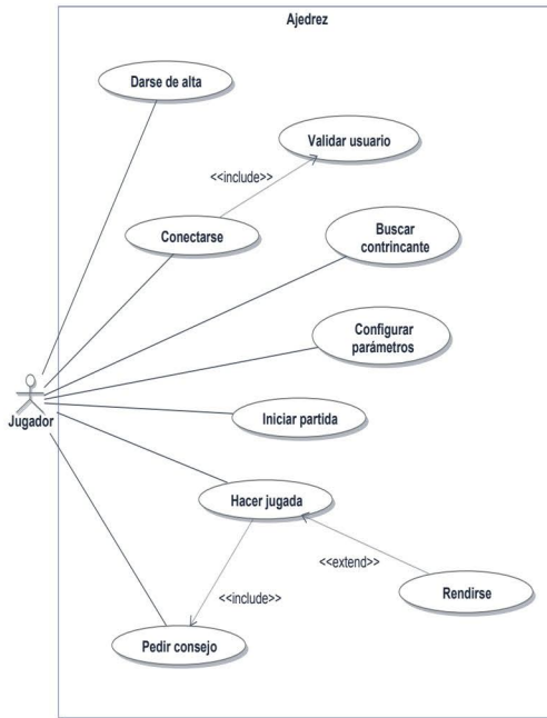
Figura 2.5. Diagrama completo con el uso de «extend»
