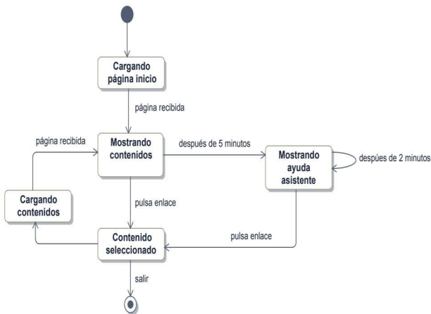
Figura 10.10. Ejemplo de diagrama de estados con dos eventos de tiempo
