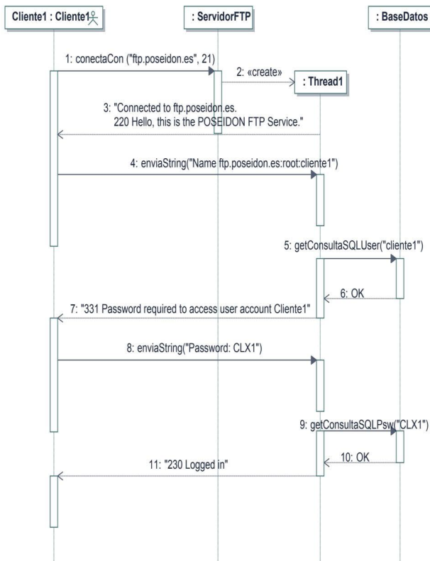
Figura 7.7. Conexión con servidor FTP usando un cliente
