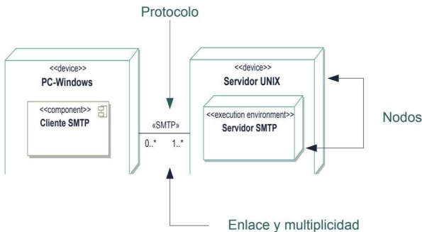
Figura 5.13. Diagrama de despliegue
