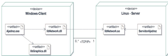
Figura 5.15. Diagrama de despliegue para el juego de ajedrez en C++
