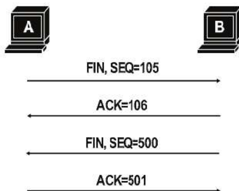
Fig. 1-54 Finalización de conexión en TCP.
