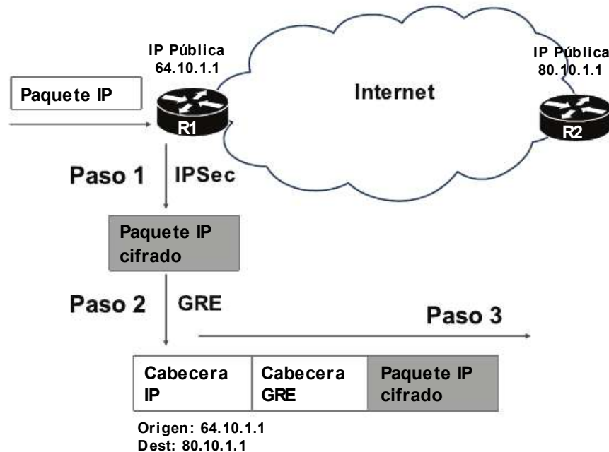
Fig. 9-4 Encapsulado GRE.
