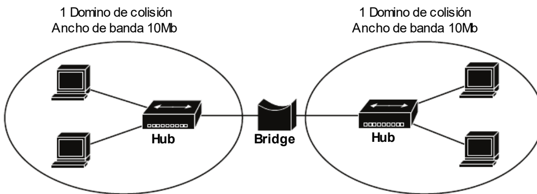
Fig. 2-1 Dominios de colisión, bridge y hub.
