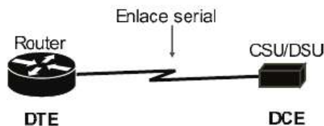
Fig. 1-38 Sincronización de enlace serial.
