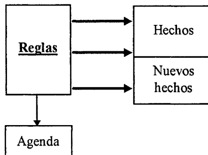
Figura 4-3 Por el método tradicional se verifica para cada regla si se cumple su antecedente a partir de la base de hechos total.
