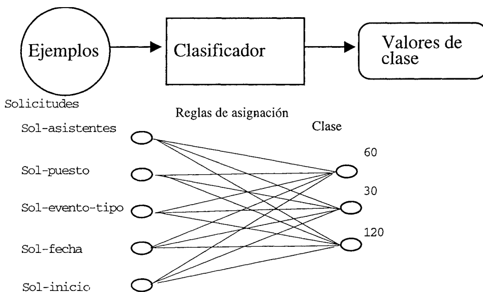
Figura 7-37 Tarea de clasificación.
