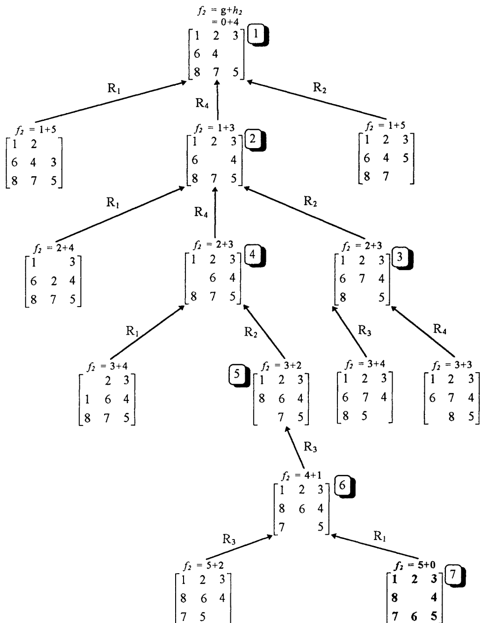
Figura 2-35 Grafo de búsqueda con h_2 .
