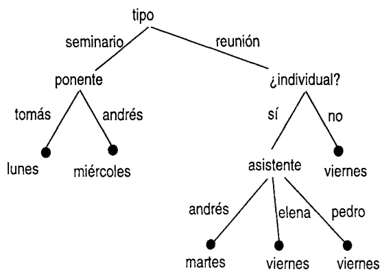
Figura 7-43 Ejemplo de árbol de decisión aprendido.
