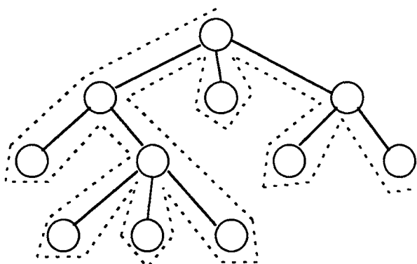
Figura 1-2 Recorrido en profundidad de izquierda a derecha de un árbol.
