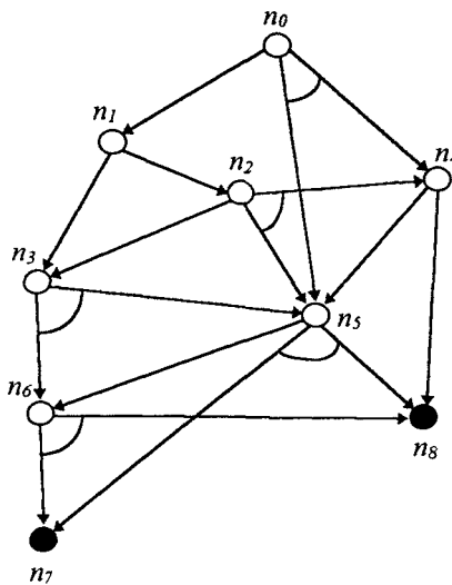
Figura 2-1 Ejemplo de grafo Y/O. Nodo inicial: n_0 . Nodos terminales: n_7 y n_8 .
