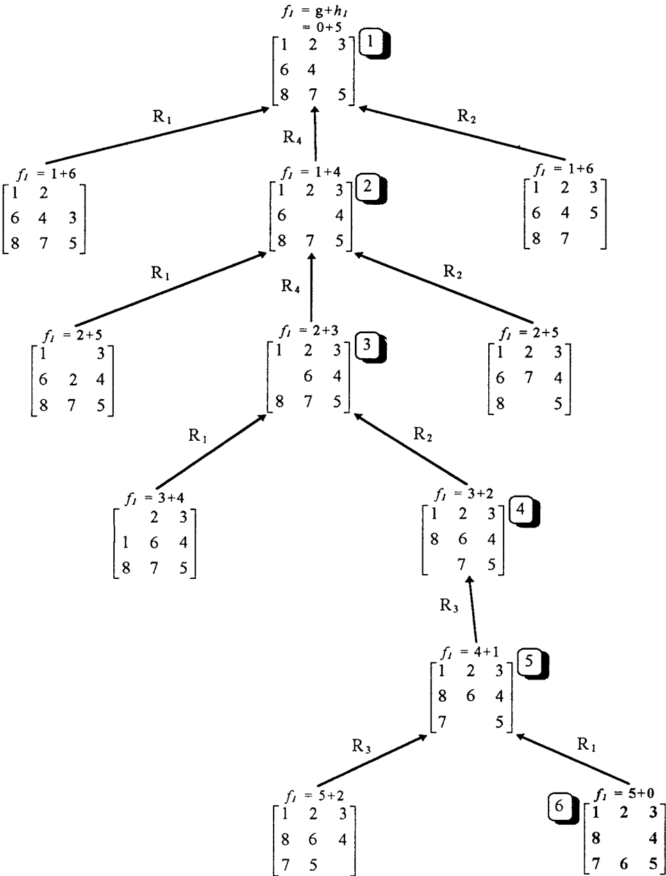
Figura 2-34 Grafo de búsqueda con h_I .
