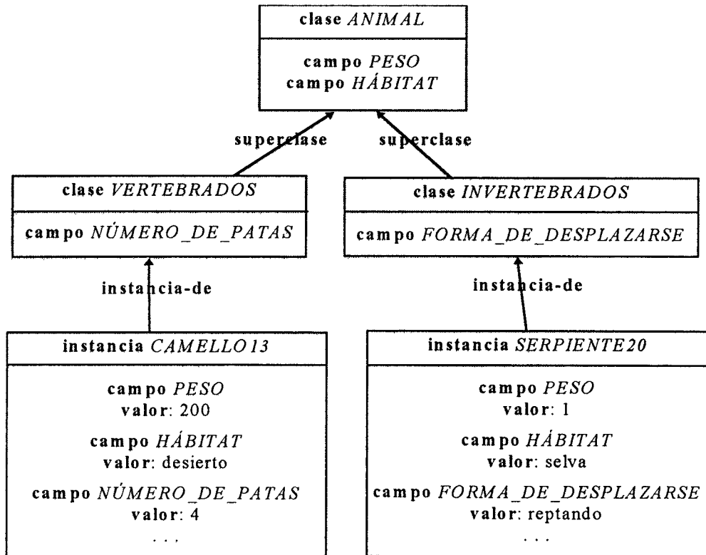
Figura 6-1 Jerarquía de marcos dotada de un mecanismo de herencia.
