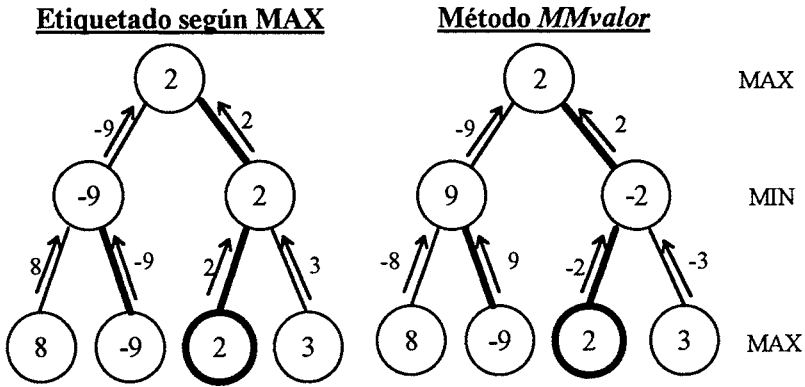
Figura 2-4 Evaluación de nodos en la estrategia MINIMAX.
