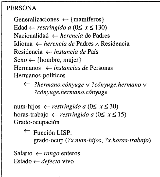
Figura 7-1 Marco genérico de Persona con diferentes formas de inferencia.
