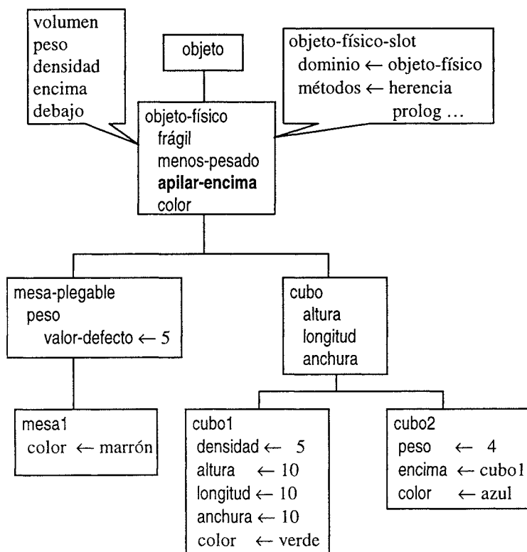
Figura 7-17 Jerarquía de relaciones entre objetos.
