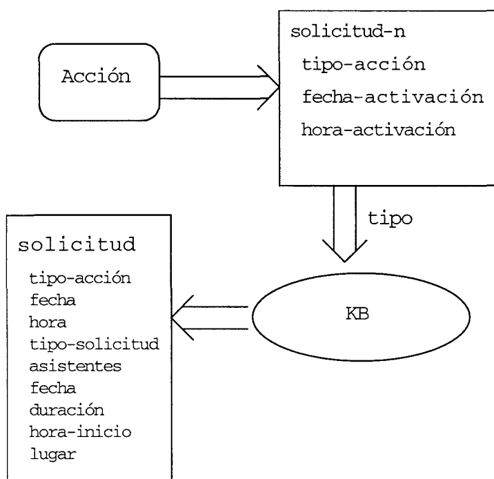
Figura 7-28 Flujo de acciones en CAP.
