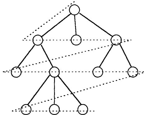
Figura 1-1 Recorrido en amplitud de izquierda a derecha de un árbol.
