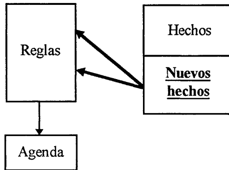
Figura 4-2 En el algoritmo RETE los nuevos hechos buscan reglas.
