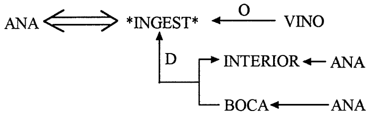
Figura 5-3 Grafo de dependencia conceptual correspondiente a la frase: “Ana bebe vino”.
