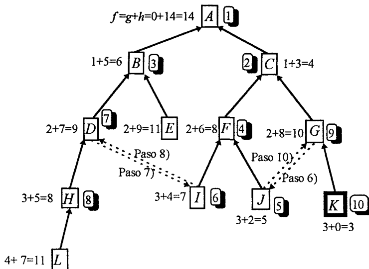
Figura 2-9 Método A*.
