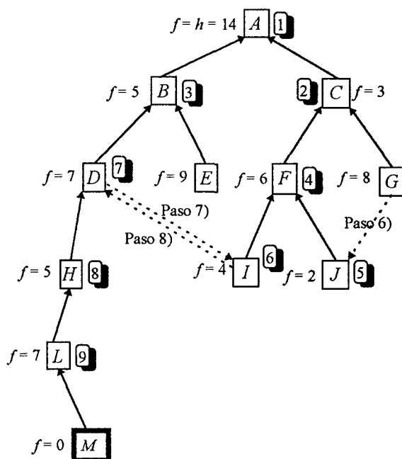
Figura 2-8 Método primero el mejor .
