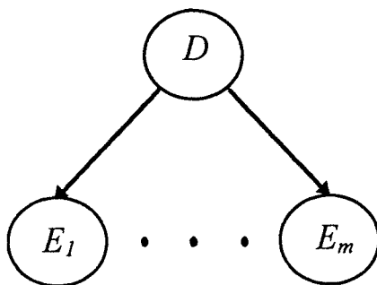
Figura 5-7 Método clásico de diagnóstico probabilista. La variable D puede tomar n valores: los n diagnósticos d_i posibles.
