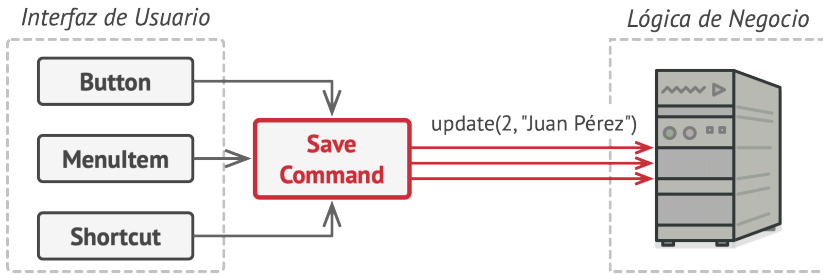
Acceso a la capa de lógica de negocio a través de un comando.
