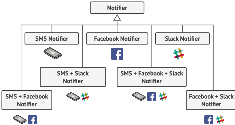
Explosión combinatoria de subclases.
