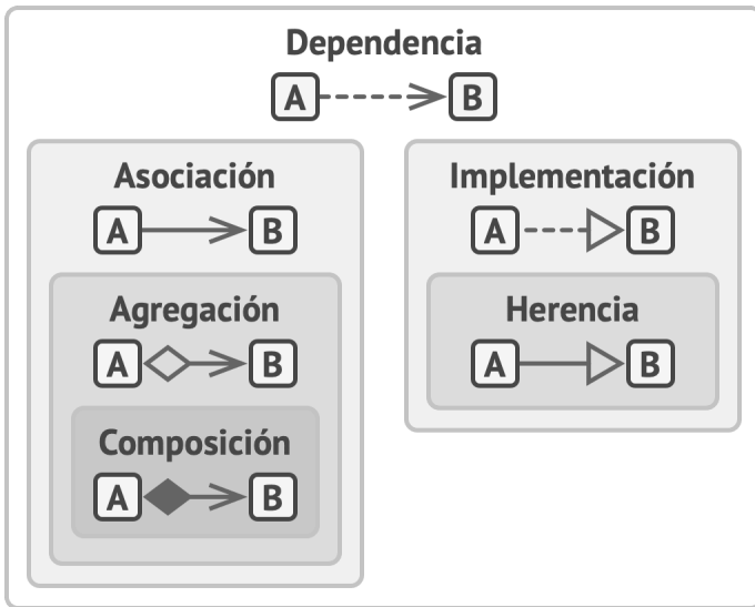
Relaciones entre objetos y clases: de la más débil a la más fuerte.
