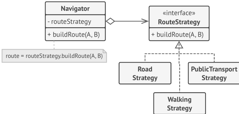
Estrategias de planificación de rutas.
