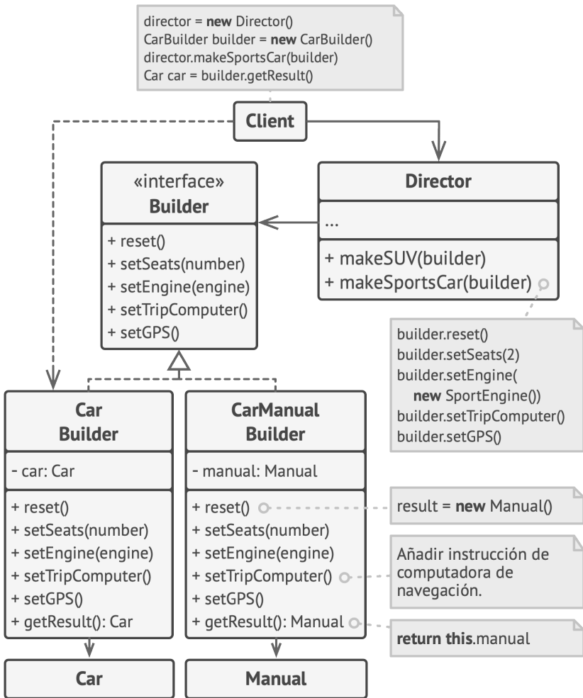
Ejemplo de una construcción paso a paso de automóviles y de los manuales de usuario para esos modelos de automóvil.
