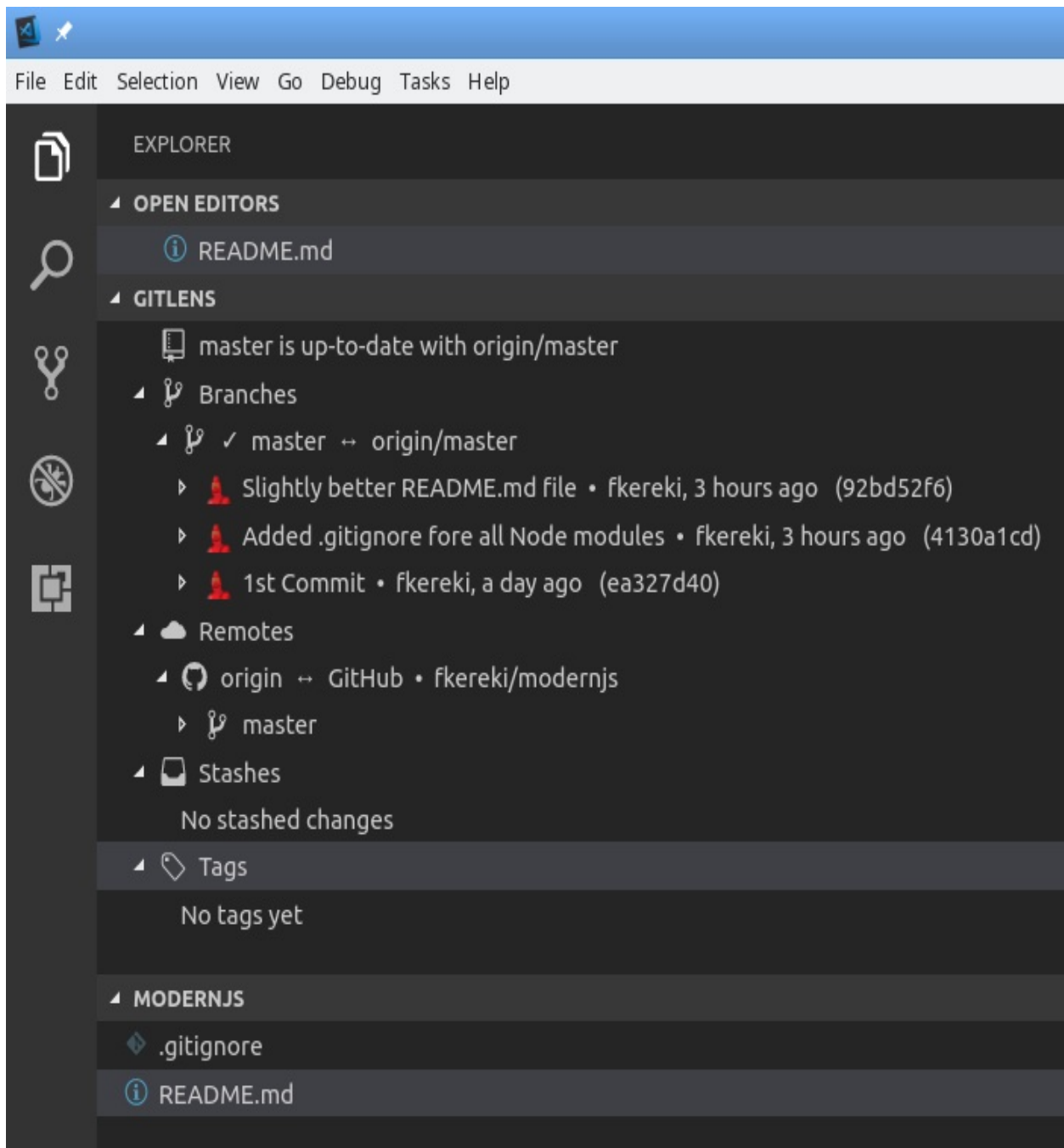
GitLens in use
