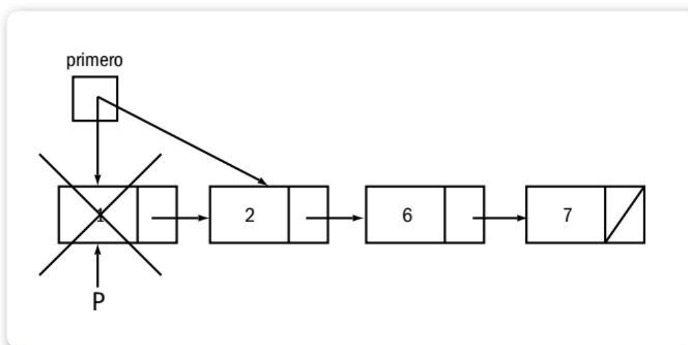
Figura 27. Esta imagen nos muestra lo que sucede si eliminamos el primer nodo.
