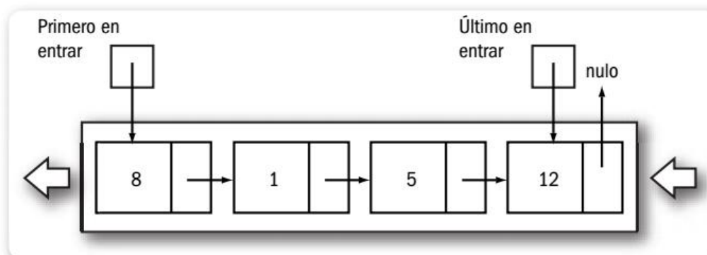
► Figura 48. Representación del funcionamiento de una cola y los diferentes elementos que debemos tener en cuenta.
