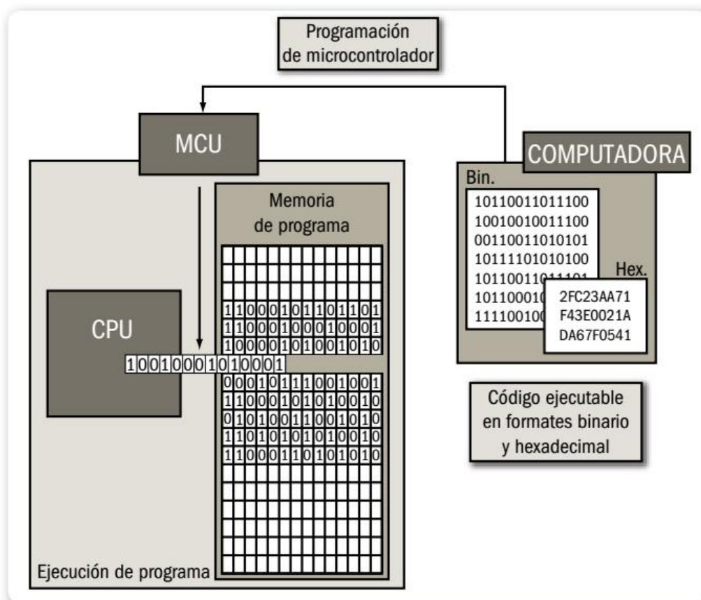
► Figura 10. Interpretación general de cómo se vería la comunicación de instrucciones al procesador.
