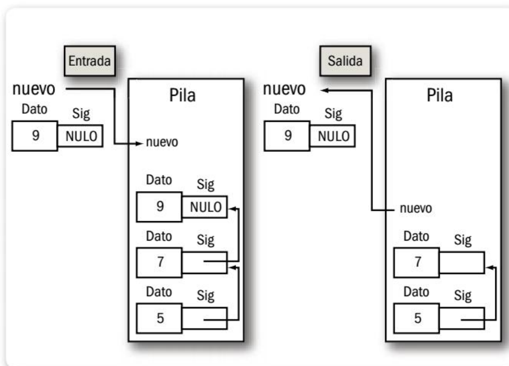
► Figura 43. Representación gráfica de lo que sucede al insertar y eliminar en una pila.
