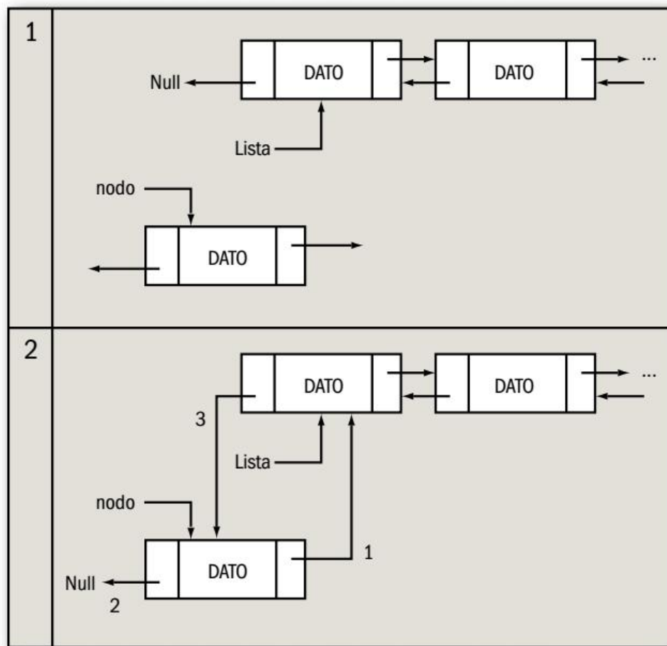
► Figura 33. Representación de lo que sucede en una lista doblemente enlazada al ejecutar los pasos vistos antes.
