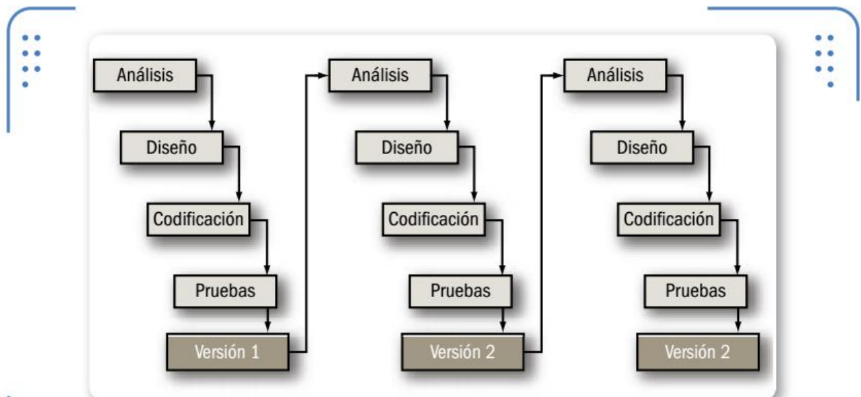
► Figura 7. Modelo iterativo. Estas iteraciones se repiten hasta obtener un producto que satisfaga las necesidades del cliente.
