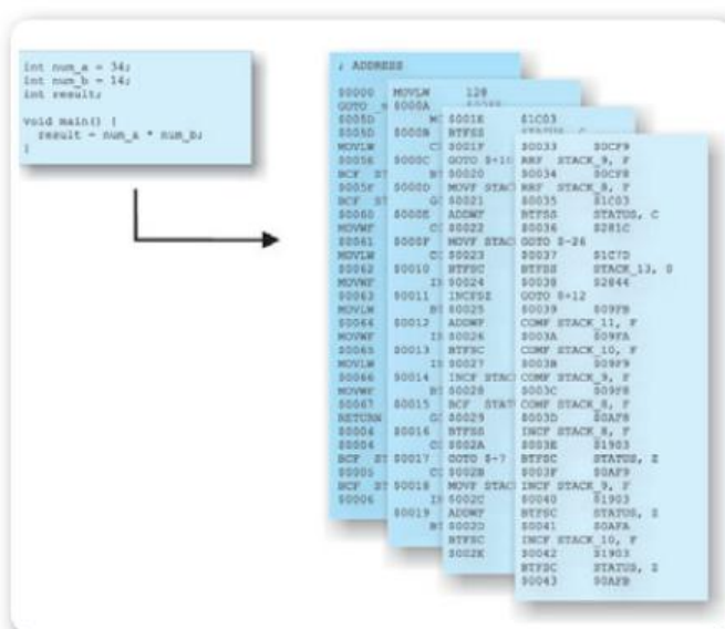
► Figura 11. El código fuente de la izquierda representa el código en lenguaje C; y el de la derecha, el código en ASSEMBLER.
