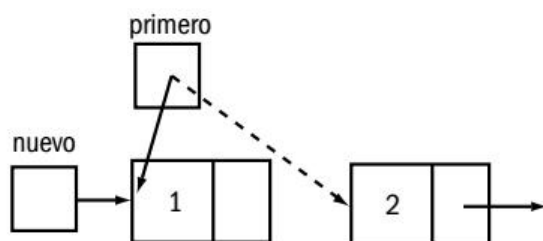
Figura 22. Aquí se representa si el valor que se ingresa es menor que el primer nodo, y cómo sería la asignación del puntero.
