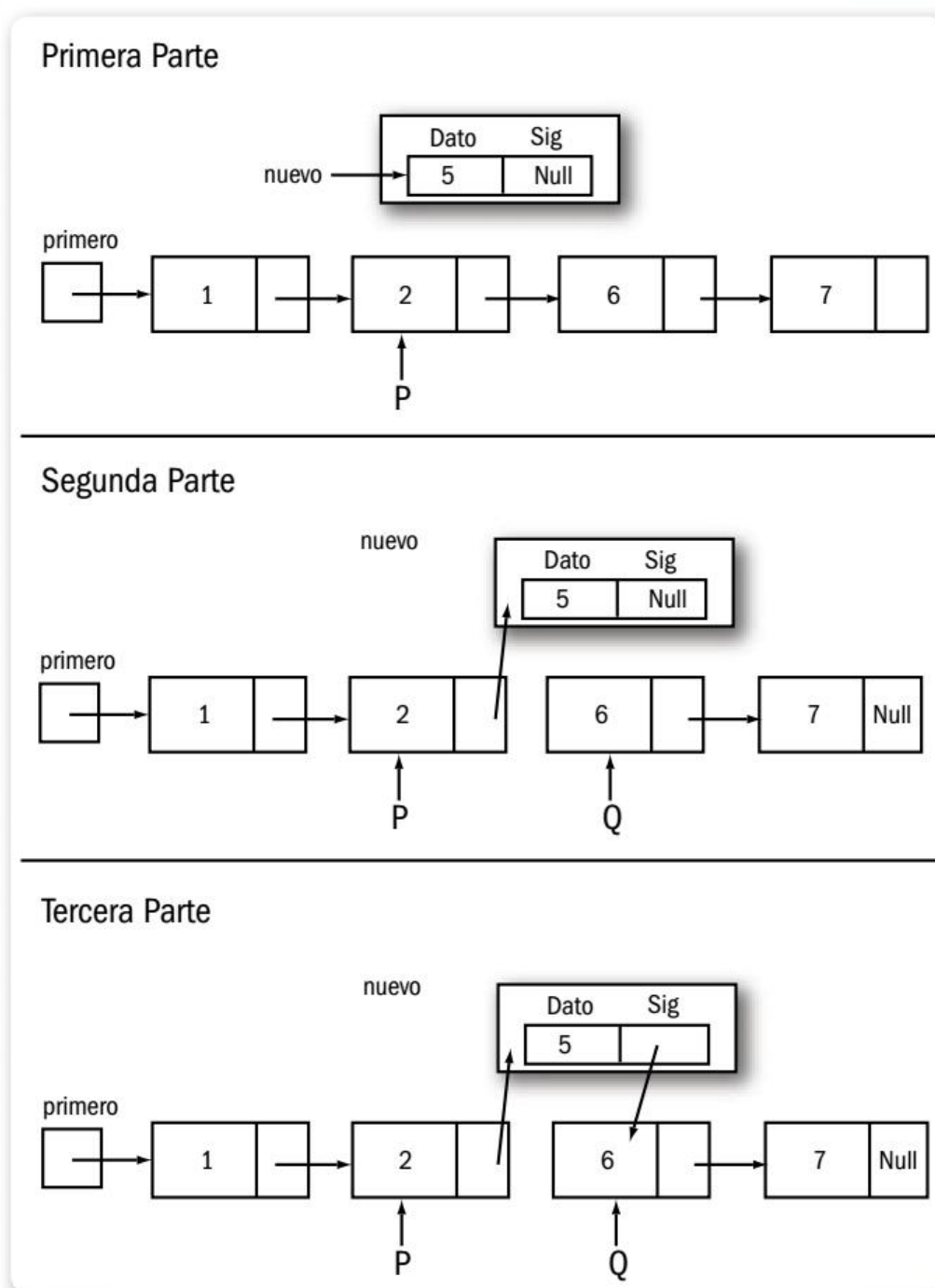
Figura 23. Representación en tres partes de cómo funciona la inserción entre nodos.
