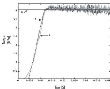
Fig. 2.174 Par para un ángulo de 0° (A), 30° (B) y la referencia (C).
