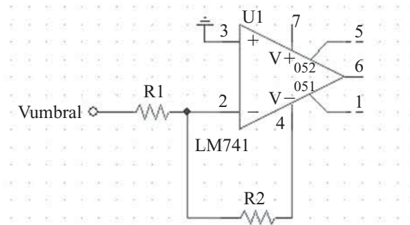
Fig. 3.23 Configuración con inversor de ganancia unitario.
