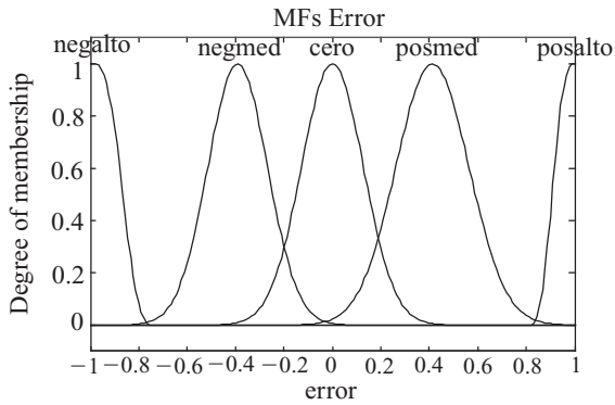
Fig. 2.93 Funciones de membresía del error.
