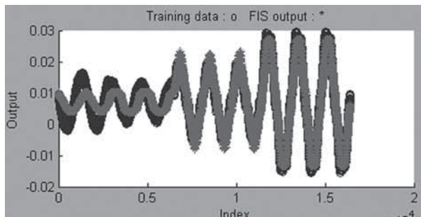
Fig. 3.90 Entrenamiento del ANFIS.
