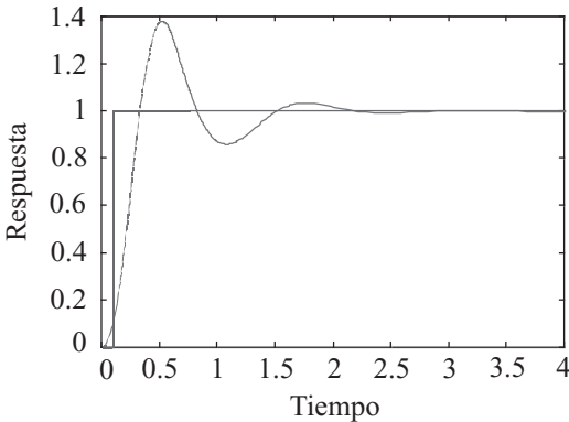
Fig. 2.90 Respuesta con el controlador 8.
