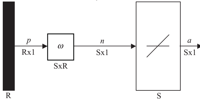
Fig. 3.44 Estructura de un asociador lineal.
