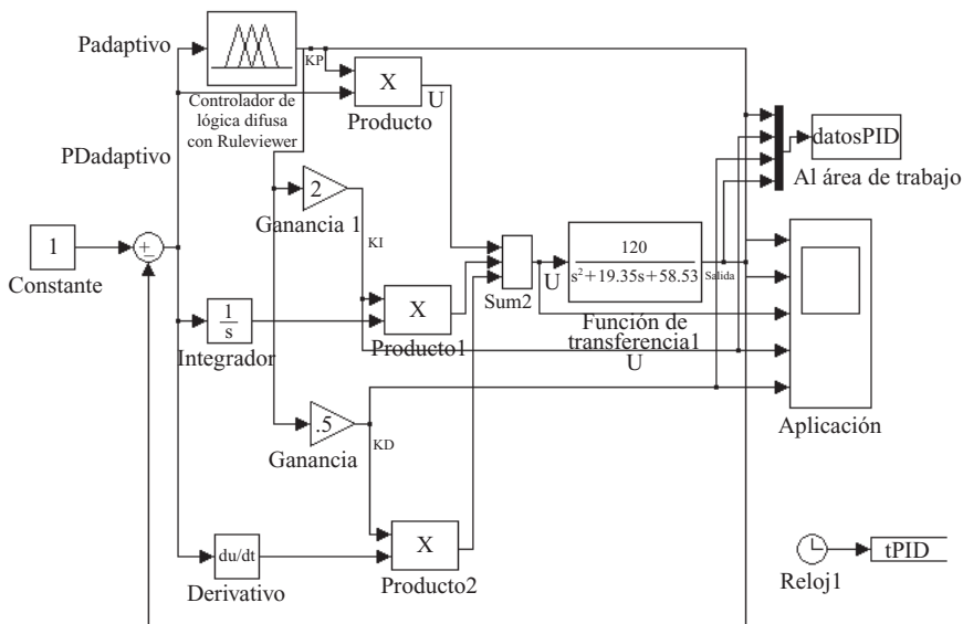
Fig. 2.113 Diagrama de bloques del sistema de control tipo PID mediante Ziegler-Nichols.
