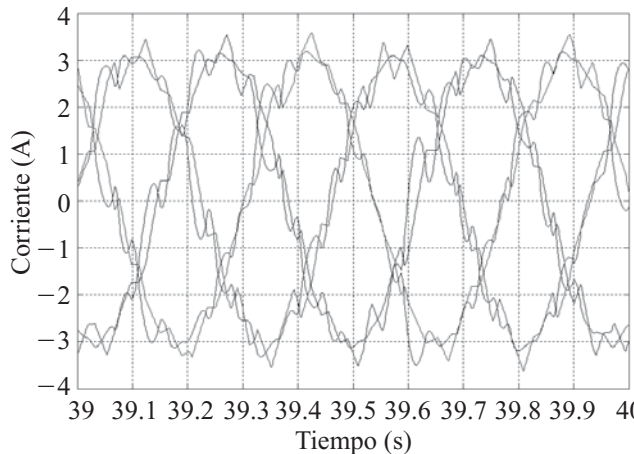
Fig. 3. 83 PWM Banda de histéresis.
