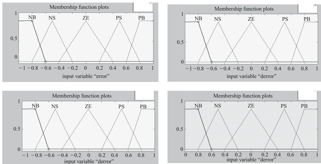
Fig. 2.88 Funciones de pertenencia para el controlador 8.
