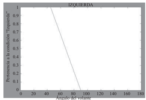
Fig. 2.22 Función hombro derecho aplicada al ángulo de un volante.
