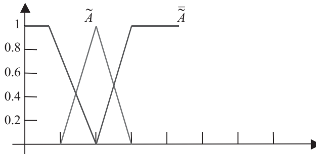
Fig. 2.7 Gráfica difusa.
