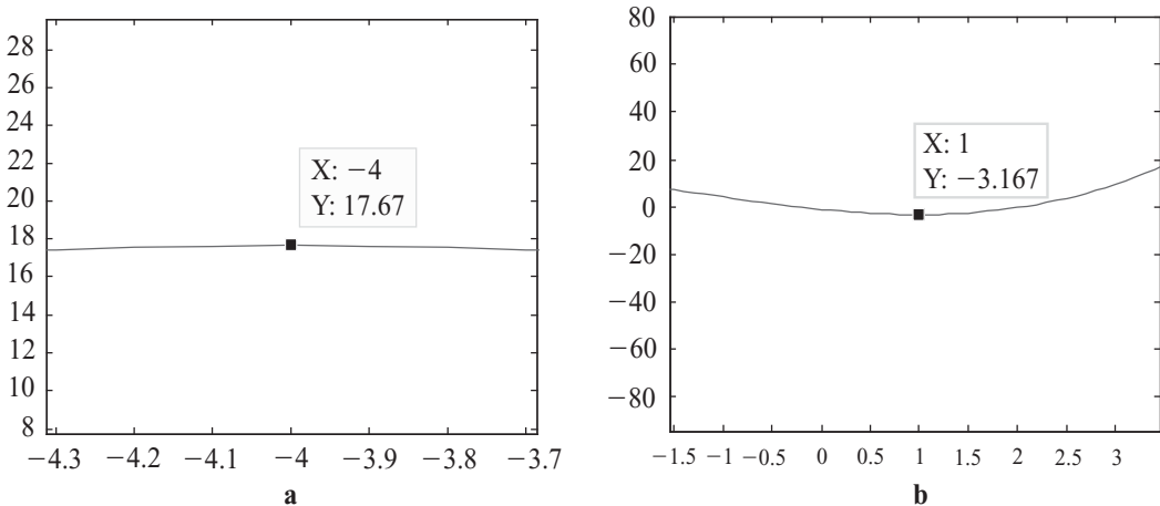
Fig. A.4 La gráfica (a) muestra el máximo de la función y (b) el mínimo.
