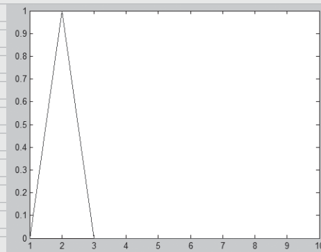
Gráfica triangular.
