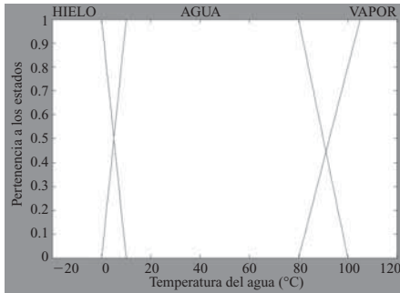
Fig. 2.28 Traslapo de las funciones de pertenencia correspondientes a los estados físicos del agua en transición.
