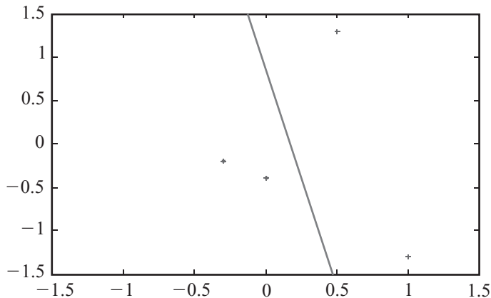
Fig. 3.14 Perceptrón entrenado.
