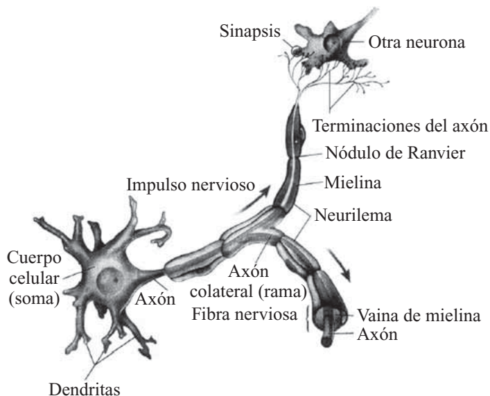
Fig. 3.1 Elementos neurales.
