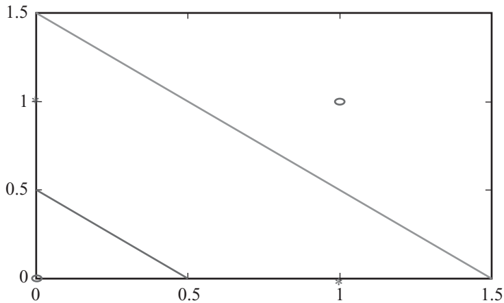
Fig. 3.18 Gráfica del XOR con clasificación.
