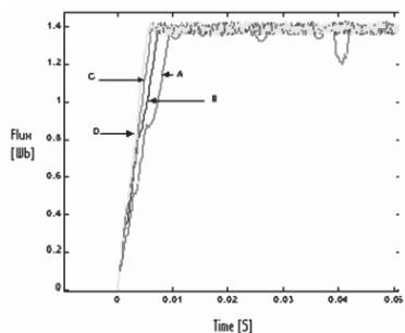
Fig. 2.175 Respuesta del flujo del estator para un ángulo de 0° (A), 15° (B), 25° (C) y 30° (D).
