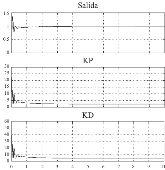
Fig. 2.112 Simulación con el controlador difuso tipo PI por Ziegler-Nichols.
