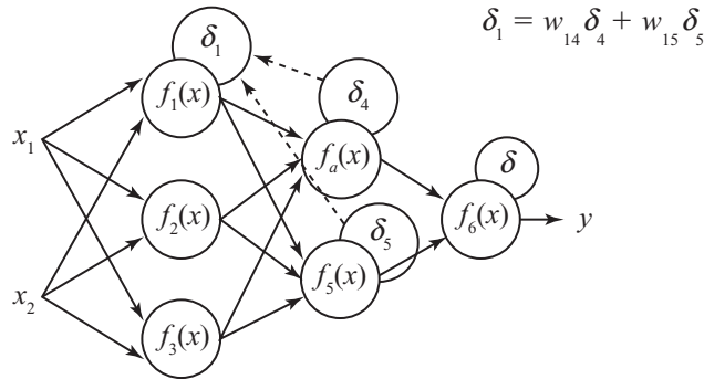
Fig. 1.9 Retropropagación del error en capas intermedias.
