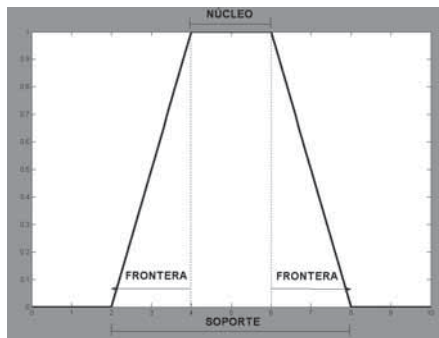
Fig. 2.29 Partes de una función de membresía.
