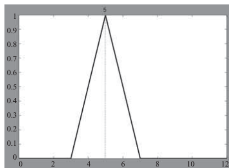
Fig. 2.32 Número difuso 5.
