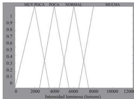
Fig. 2.58 Funciones de pertenencia para la intensidad luminosa.
