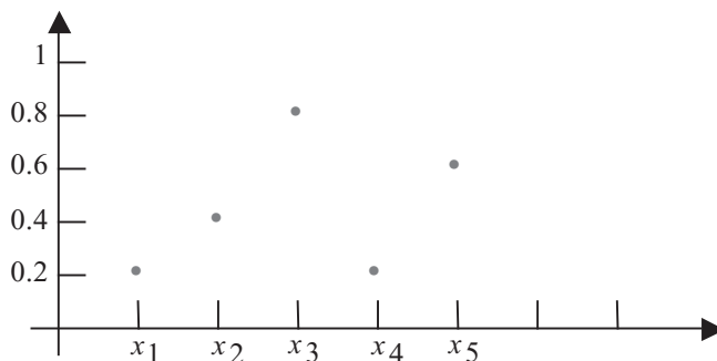
Fig. 2.5 Gráfica difusa.
