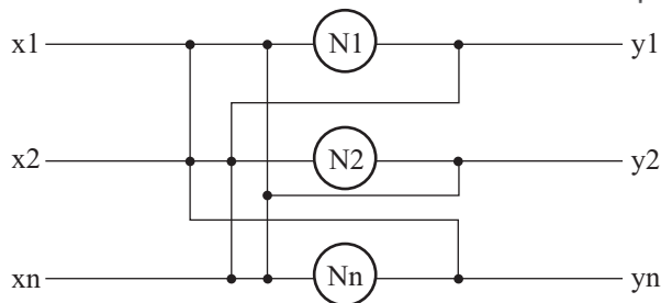
Fig. 3.48 Red Hopfield.
