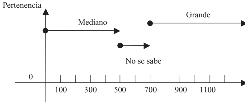
Fig. 2.2 Gráfica de valores numéricos en un conjunto semi-nítido.
