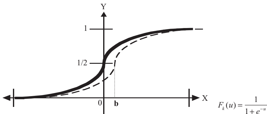
Fig. 3.5 Función sigmoideal.
