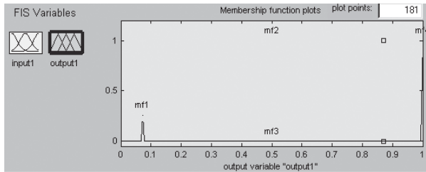
Fig. 2.121 Salida Singleton.
