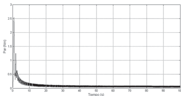
Fig. 3. 80 Par electromagnético.
