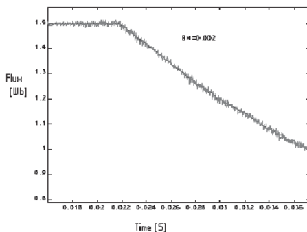
Fig. 2.176 Respuesta del flujo del estator en par constante y regiones de debilitamiento del campo para un ángulo de 300° y H_B=0.002 .
