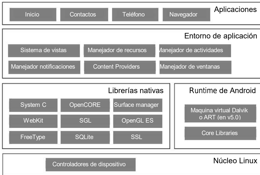
Figura 2: Arquitectura de Android.
