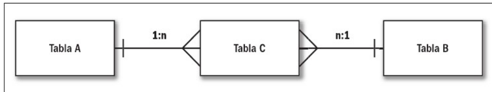
Figura 18. Transformación de relaciones varios a varios.
