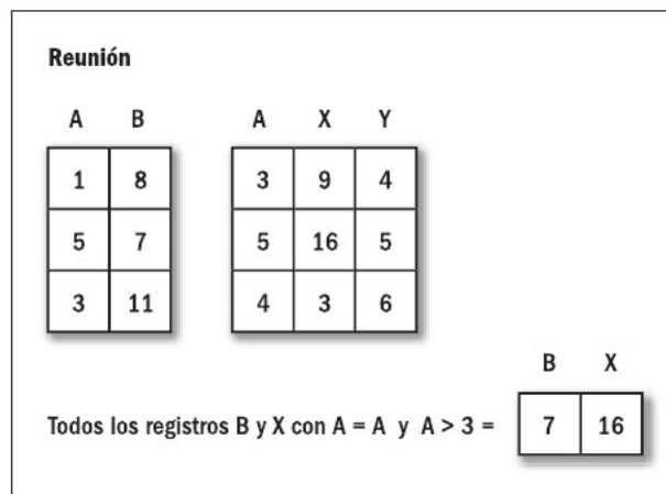
Figura 11. Reunión.
