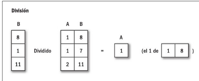
Figura 12. División.
