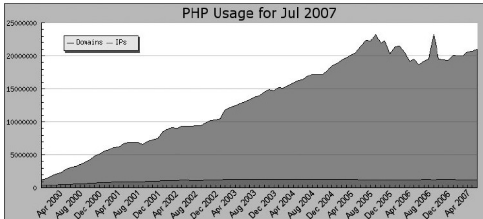
Figura 2. Uso de PHP en servidores a través del tiempo. (Fuente: http://news.netcraft.com ).
