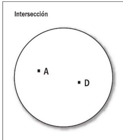
Figura 6. Intersección.
