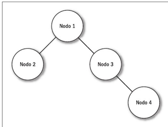
Figura 1. Modelo jerárquico.
