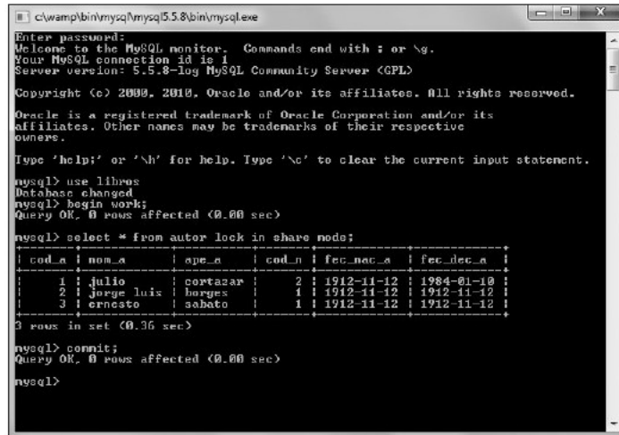
Figura 2. Finalización de una transacción a través de COMMIT.
