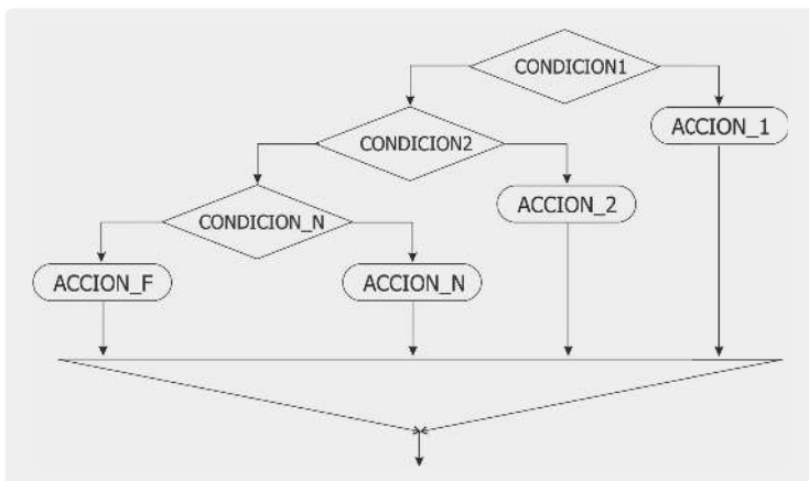
Fig. 4.1 Condicional If doblemente enlazada
