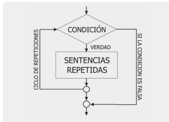
Fig. 5.1 Estructura repetitiva while
