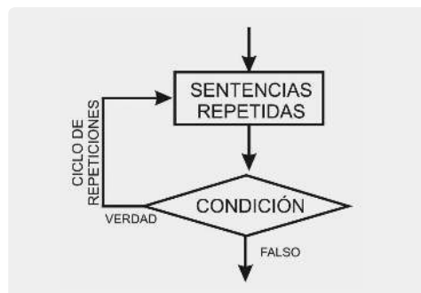
Fig. 5.3 Estructura repetitiva do...while
