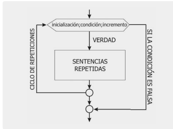
Fig. 5.2 Estructura repetitiva for
