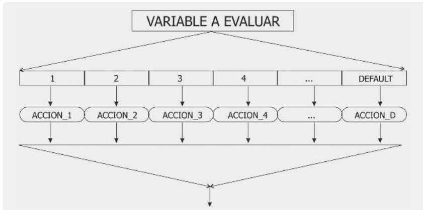
Fig. 4.1 Sentencia múltiple switch
