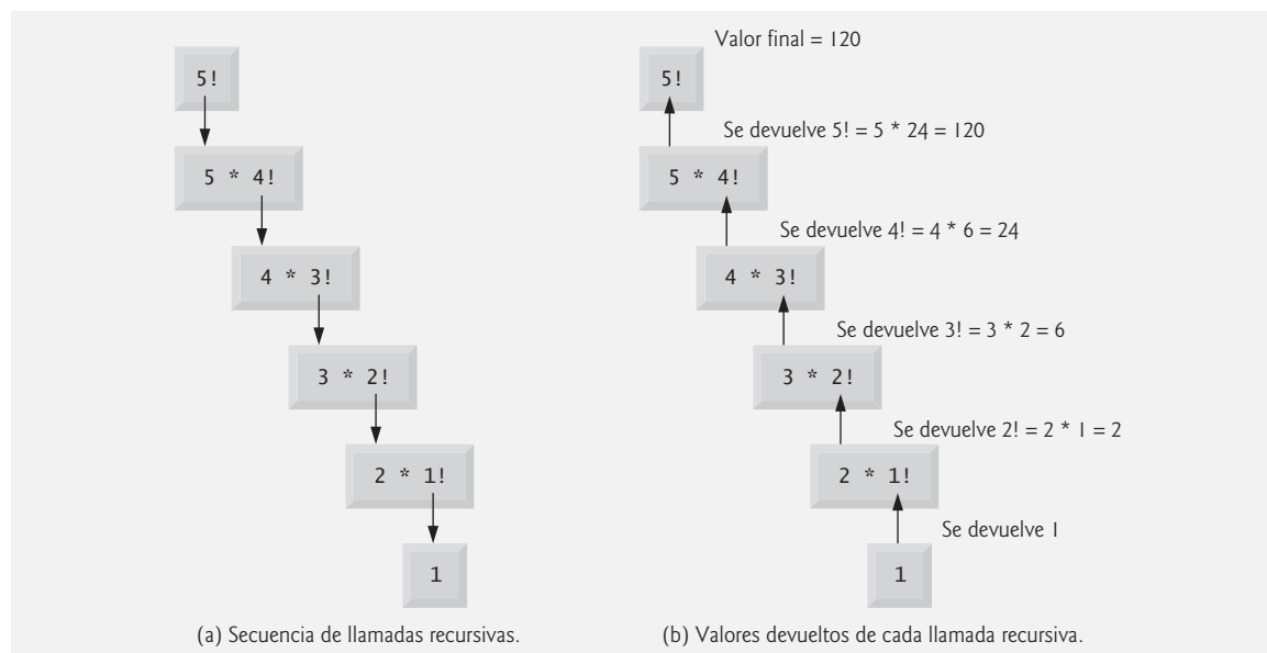
Figura 7.15 | Evaluación recursiva de 5!
