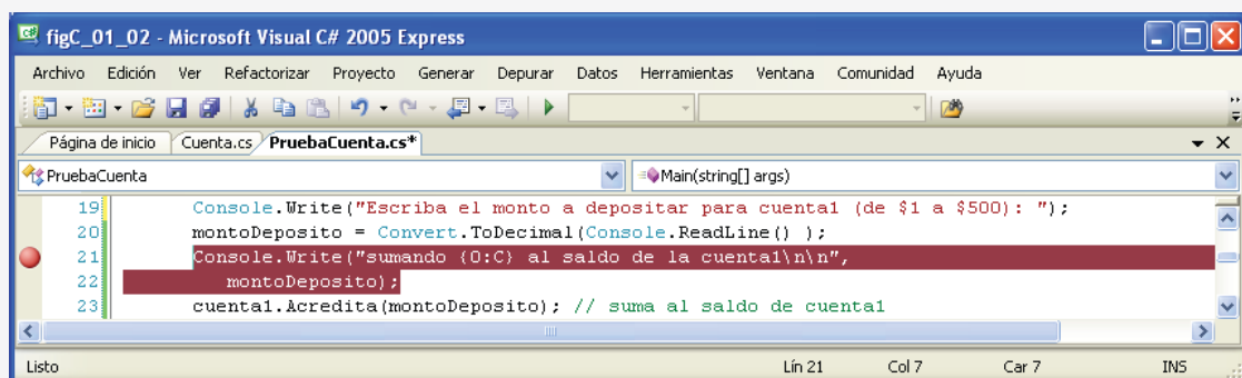
Figura C.25 | Establecimiento de un punto de interrupción en la línea 21.
