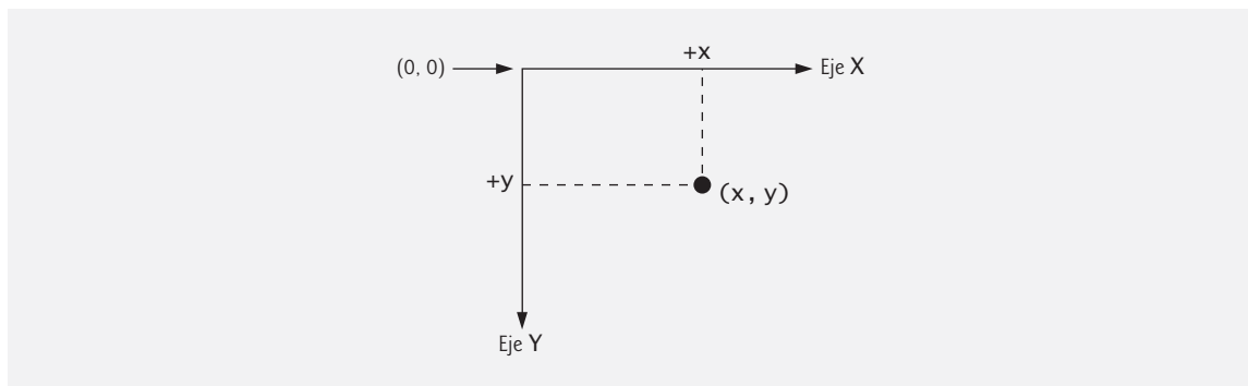
Figura 17.2 | Sistema de coordenadas de la GDI+. Las unidades se miden en píxeles.
