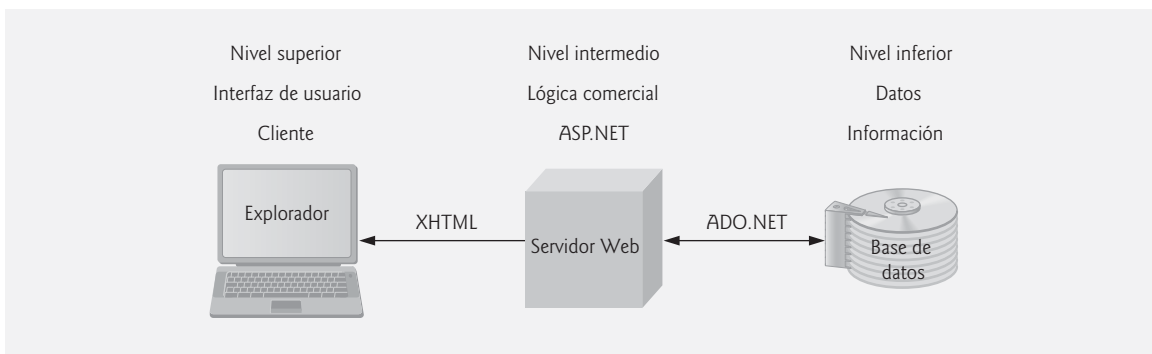
Figura 21.3 | Arquitectura de tres niveles.
