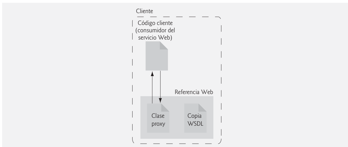
Figura 22.6 | Cliente de un servicio Web .NET, después de agregar una referencia Web.
