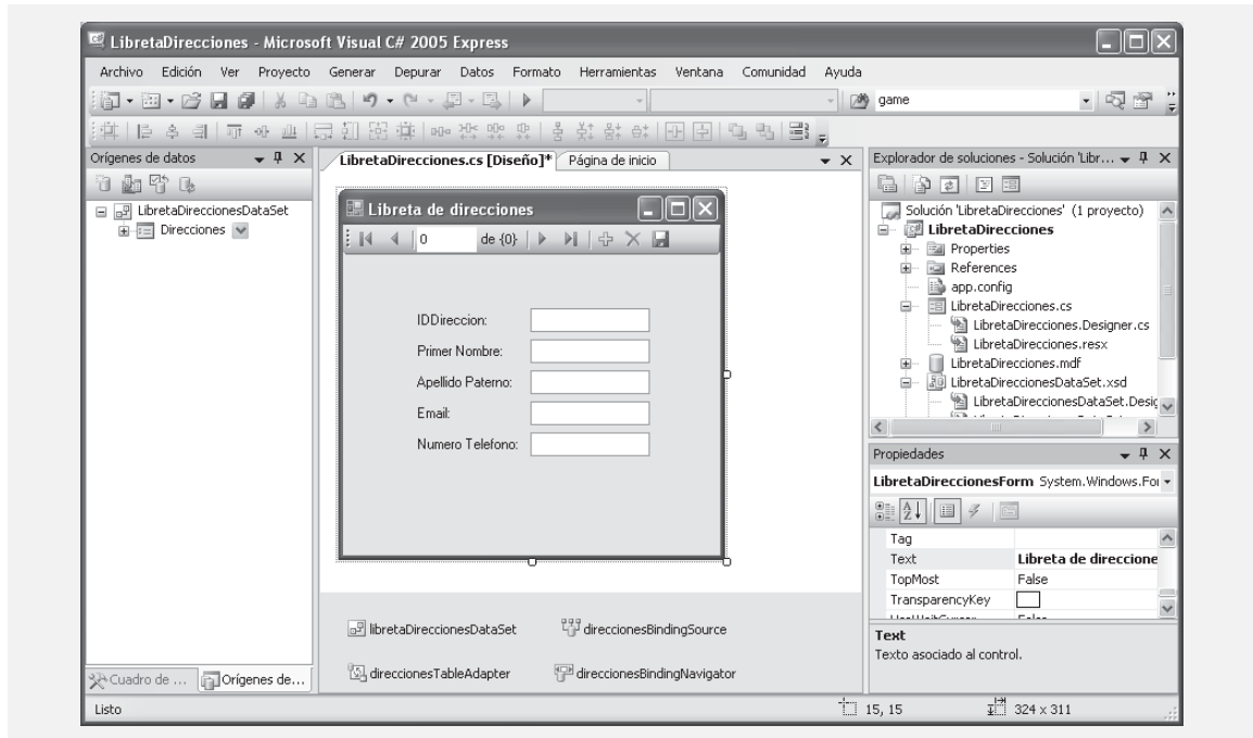
Figura 20.46 | Mostrar una tabla en un formulario, usando una serie de controles Label y TextBox.
