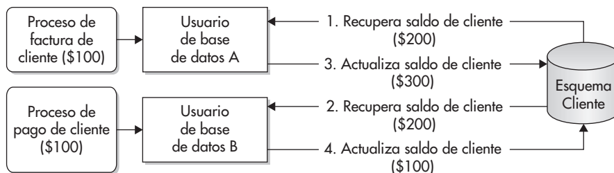
Figura 11-1 El problema de una actualización concurrente.
