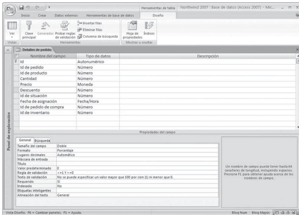
Figura 2-12 Panel de definición de la tabla Detalles de pedido, columna Descuento.
