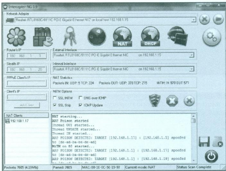
Fig. 7.5.- Interceptor-NG.
