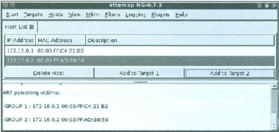
Fig. 8.15.- ARP Poisoning
