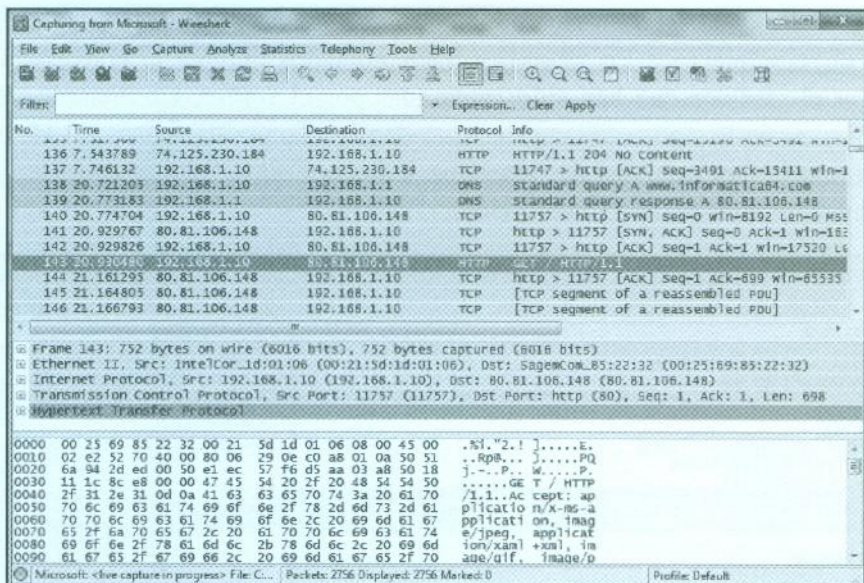
Fig. 3.3.- Wireshark.
