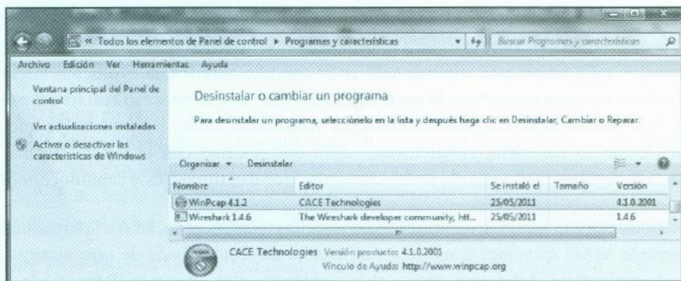
Fig. 3.2.- WinPcap.
