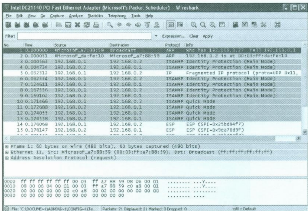
Fig. 8.7.- Comunicación ISAKMP.
