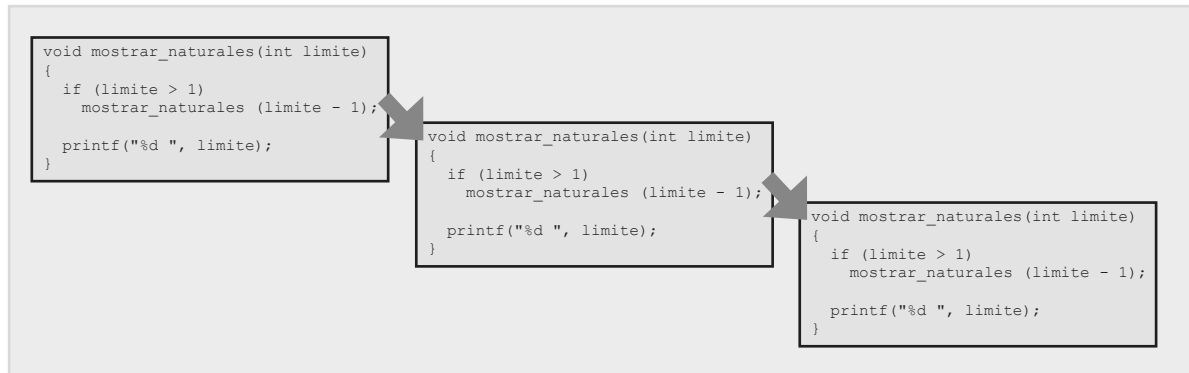
Fig. 9-3. "Anidamiento" de llamadas.
