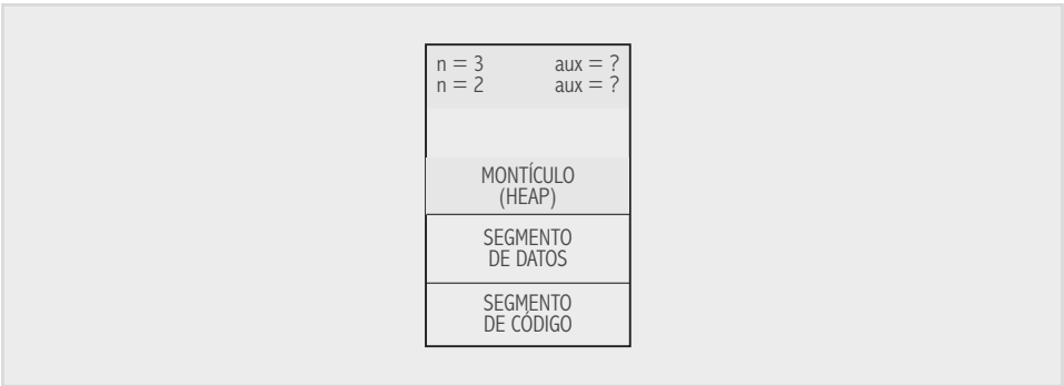
Fig. 9-6. Representación de la pila cuando se hace una llamada recursiva a factorial() .
