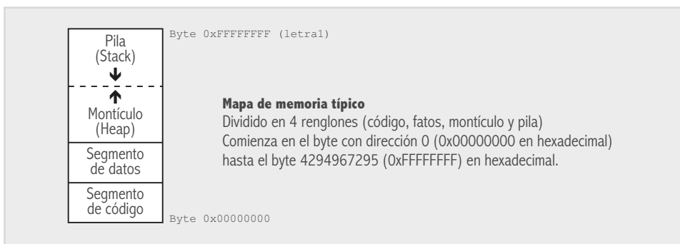
Fig. 3-5. "Regiones" de la memoria principal.
