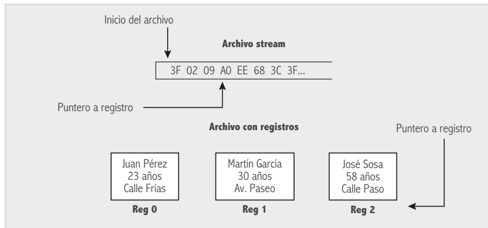
Fig. 7-2. Puntero del archivo que memoriza el byte correspondiente para una operación de lectura o escritura.
