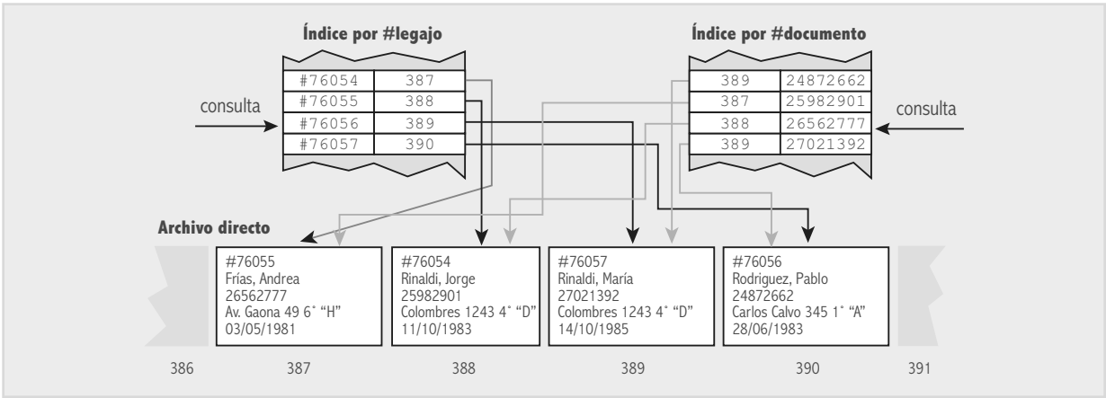
Fig. 8-3. Uso de más de un índice para acceder a un mismo conjunto de datos por medio de diferentes claves de acceso.
