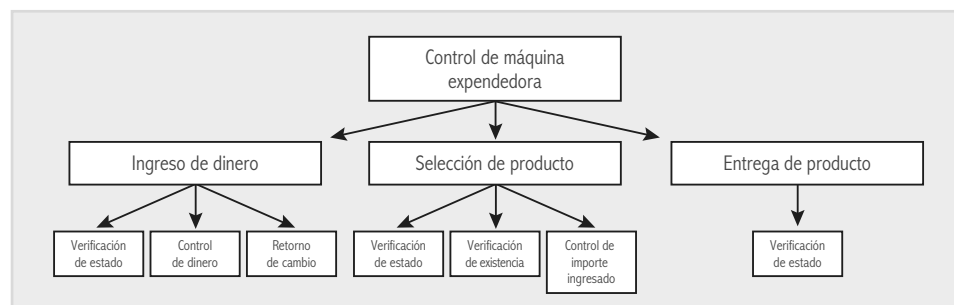
Fig. 3-1. Sistema de control de una máquina expendedora de gaseosas.
