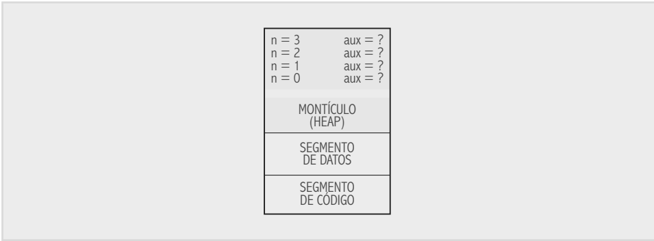
Fig. 9-8. Forma que presenta la pila con una tercer llamada recursiva.
