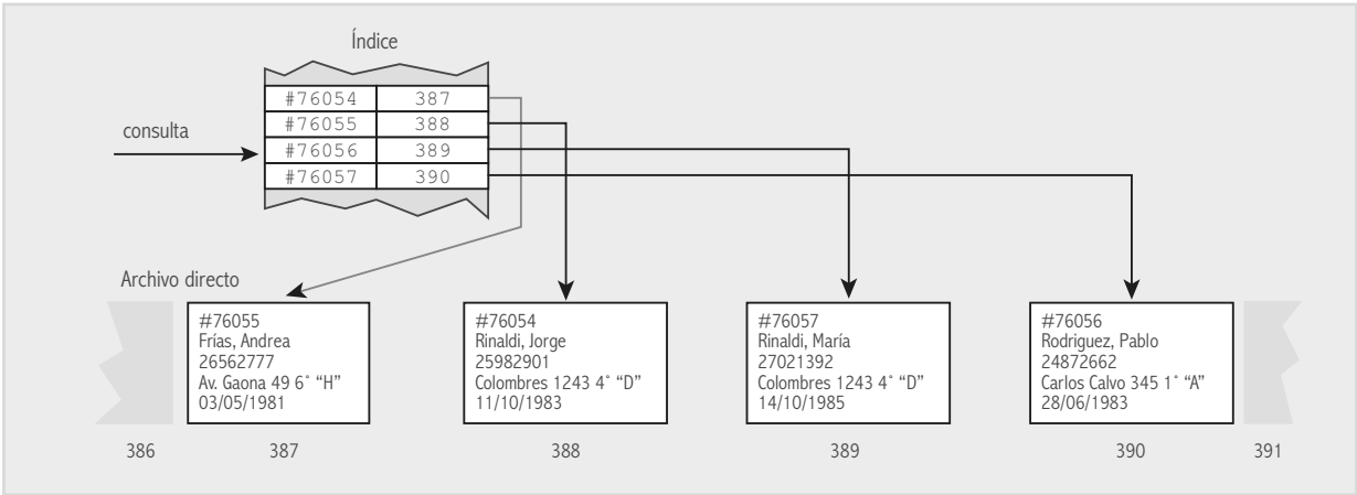
Fig. 8-2. Modo en que están organizados un archivo y su índice.
