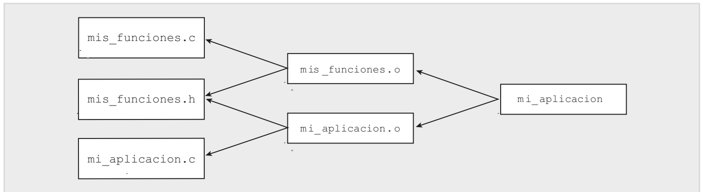
Fig. 11-5. Grafo de dependencias.
