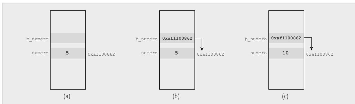
Fig. 10-4. Puntero a entero que "apunta" a la variable numero .
