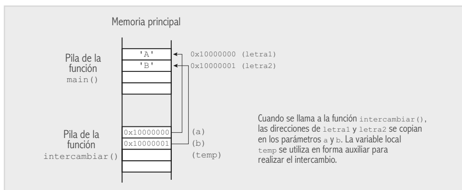
Fig. 3-2. Pasaje de parámetros en lenguaje C (pasaje por valor).
