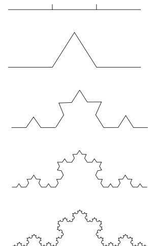
Fig. 9-2. Fractal simple (copo de nieve de Koch).
