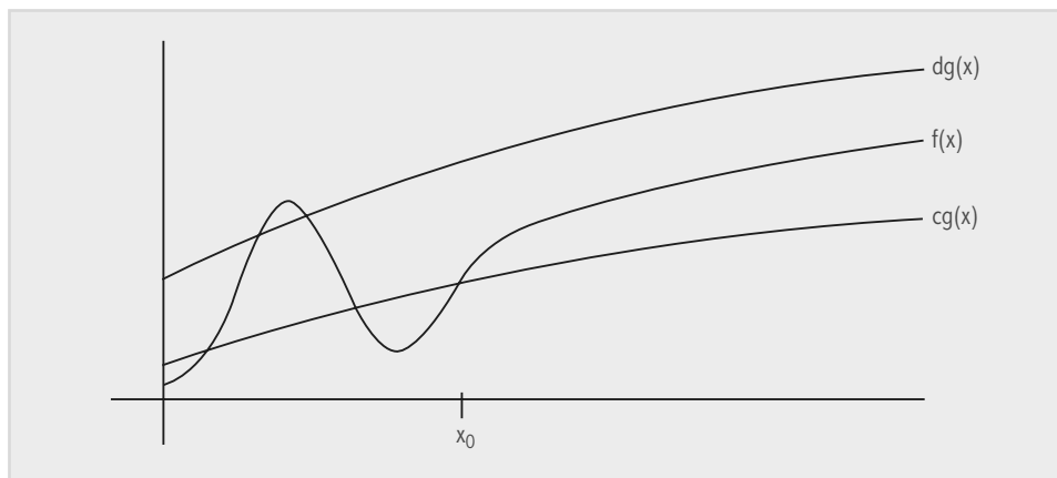
Fig. 5-3. Cota ajustada asintótica - \Theta .
