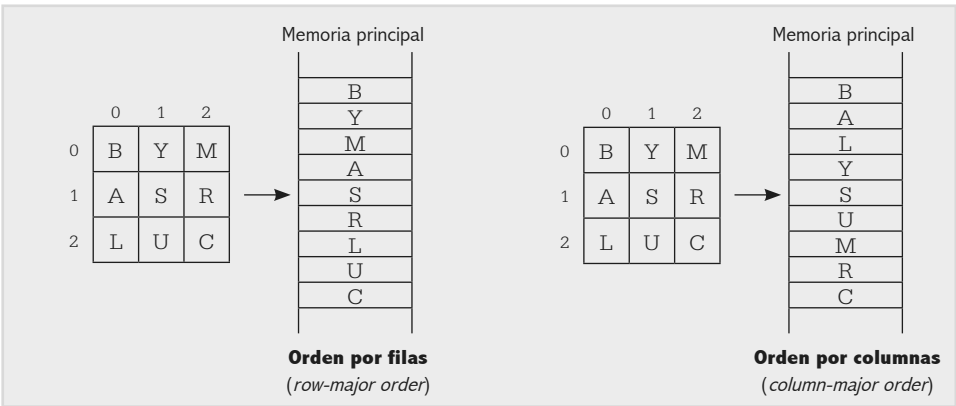
Fig. 4-4. Orden por filas (lenguajes C y Pascal) y orden por columnas (lenguaje Fortran).
