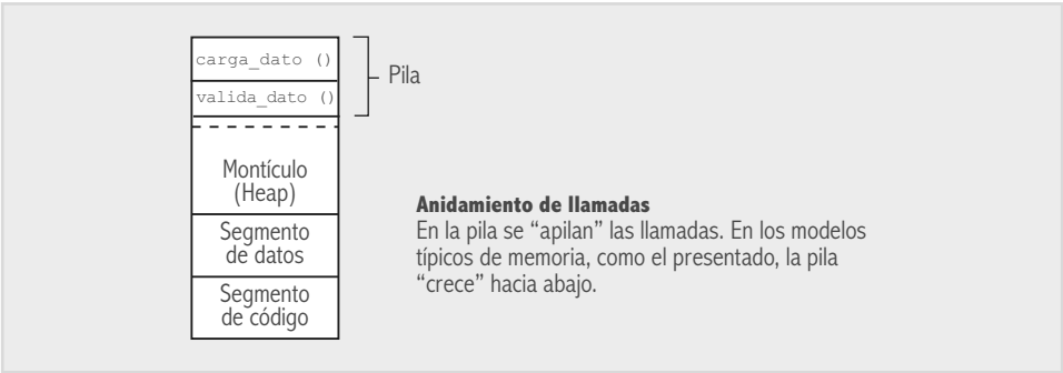
Fig. 3-6. "Anidamiento" de llamadas.
