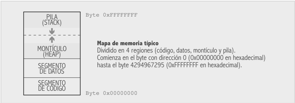
Fig. 9-4. Mapa de memoria (uso de la pila).
