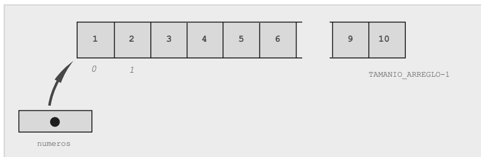
Fig. 10-5. Modo de acceder a un arreglo mediante un puntero al primer entero.
