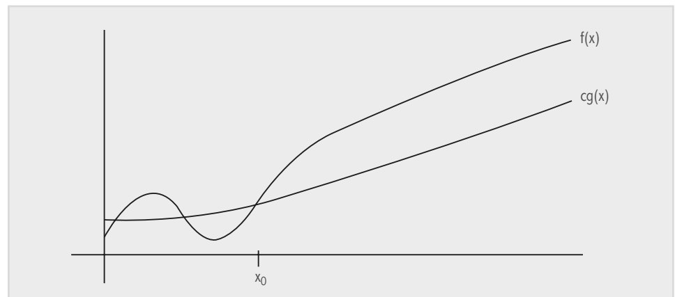
Fig. 5-2. Cota inferior asintótica - \Omega .
