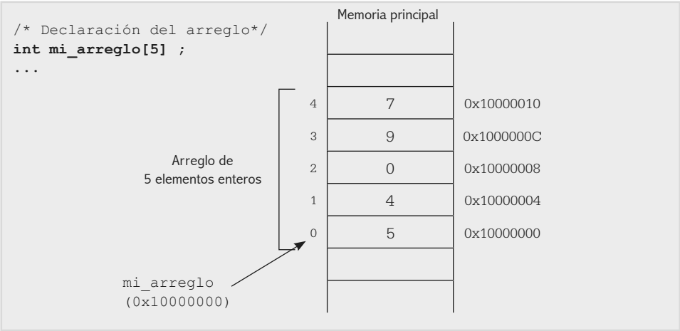
Fig. 4-5. Arreglo de 5 números enteros almacenados en memoria principal.
