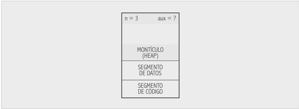
Fig. 9-5. Representación de la pila cuando se hace la primera llamada a funcion factorial() .
