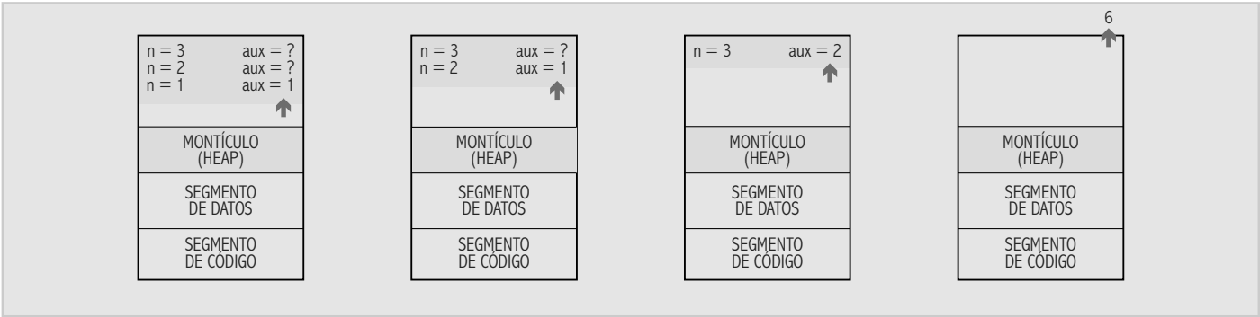
Fig. 9-9. Modo en que se “deshace” la pila en sentido inverso a como se construyó.
