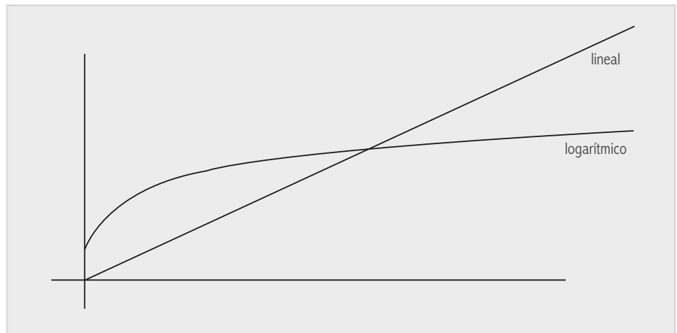
Fig. 5-4. Comparación entre búsqueda secuencial y búsqueda binaria.
