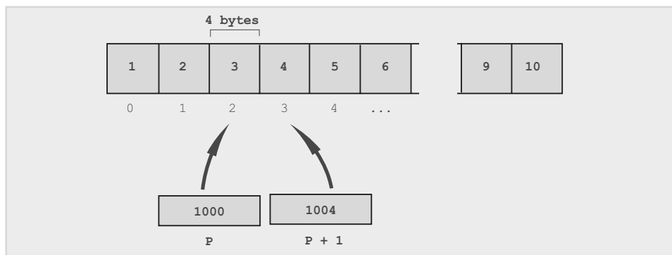
Fig. 10-6. Aplicación de operaciones aritméticas en punteros.
