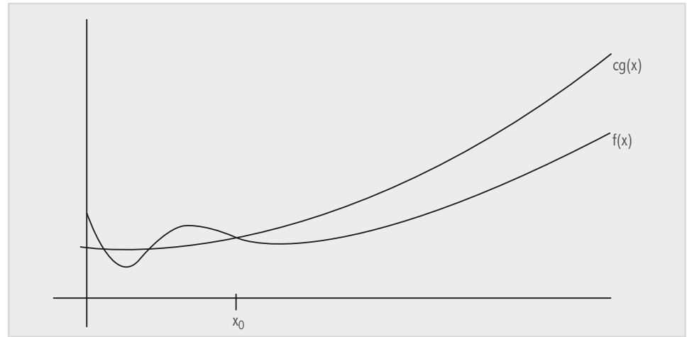
Fig. 5-1. Cota superior asintótica -O.
