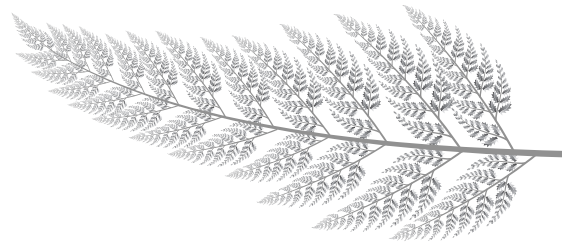
Fig. 9-1. Hoja de "helecho".
