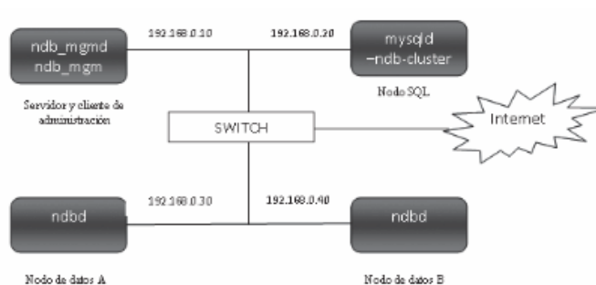
Figura 6.8. Red de equipos del cluster
